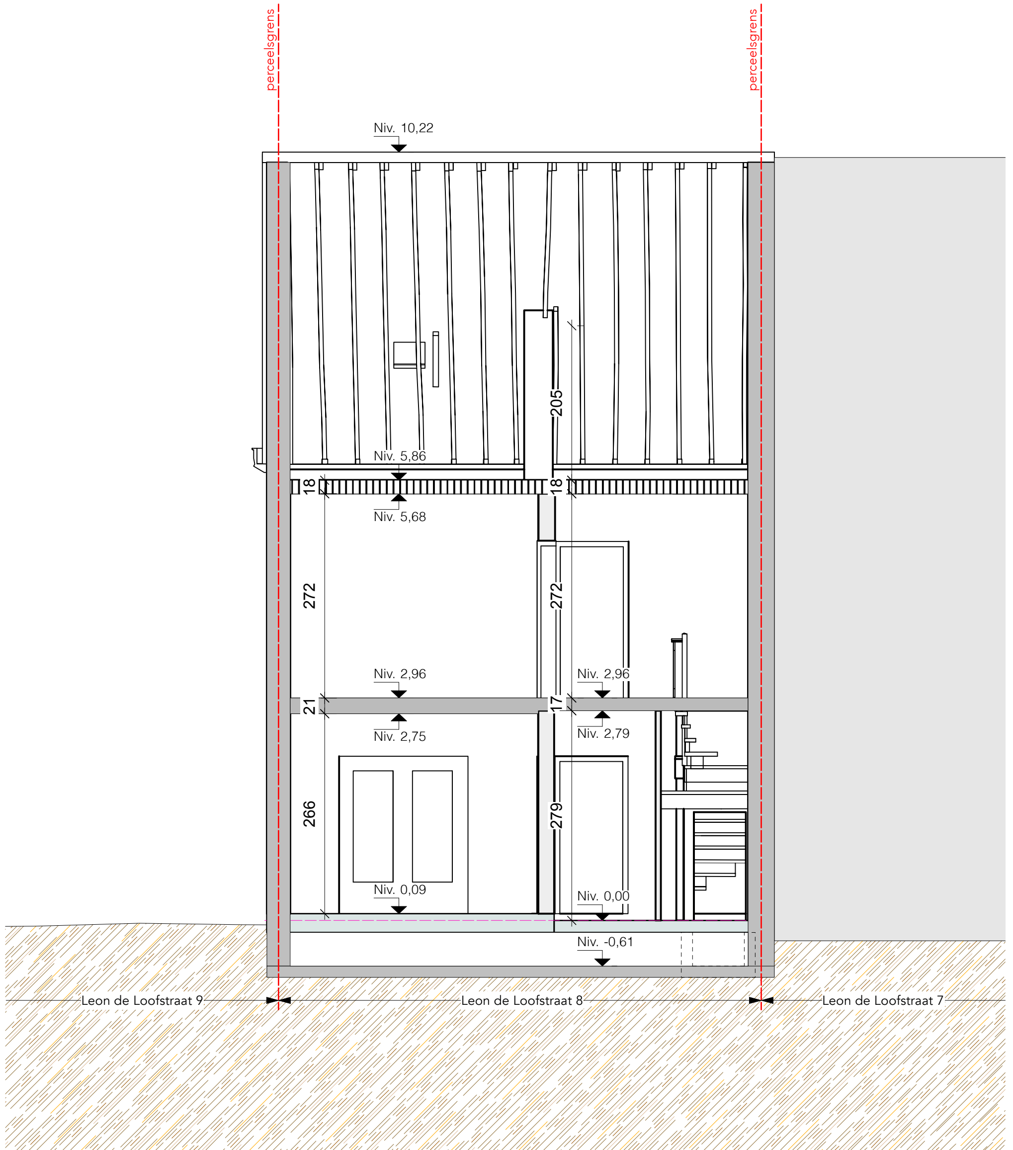
BT dwarsnede AA schaal: 1:50
