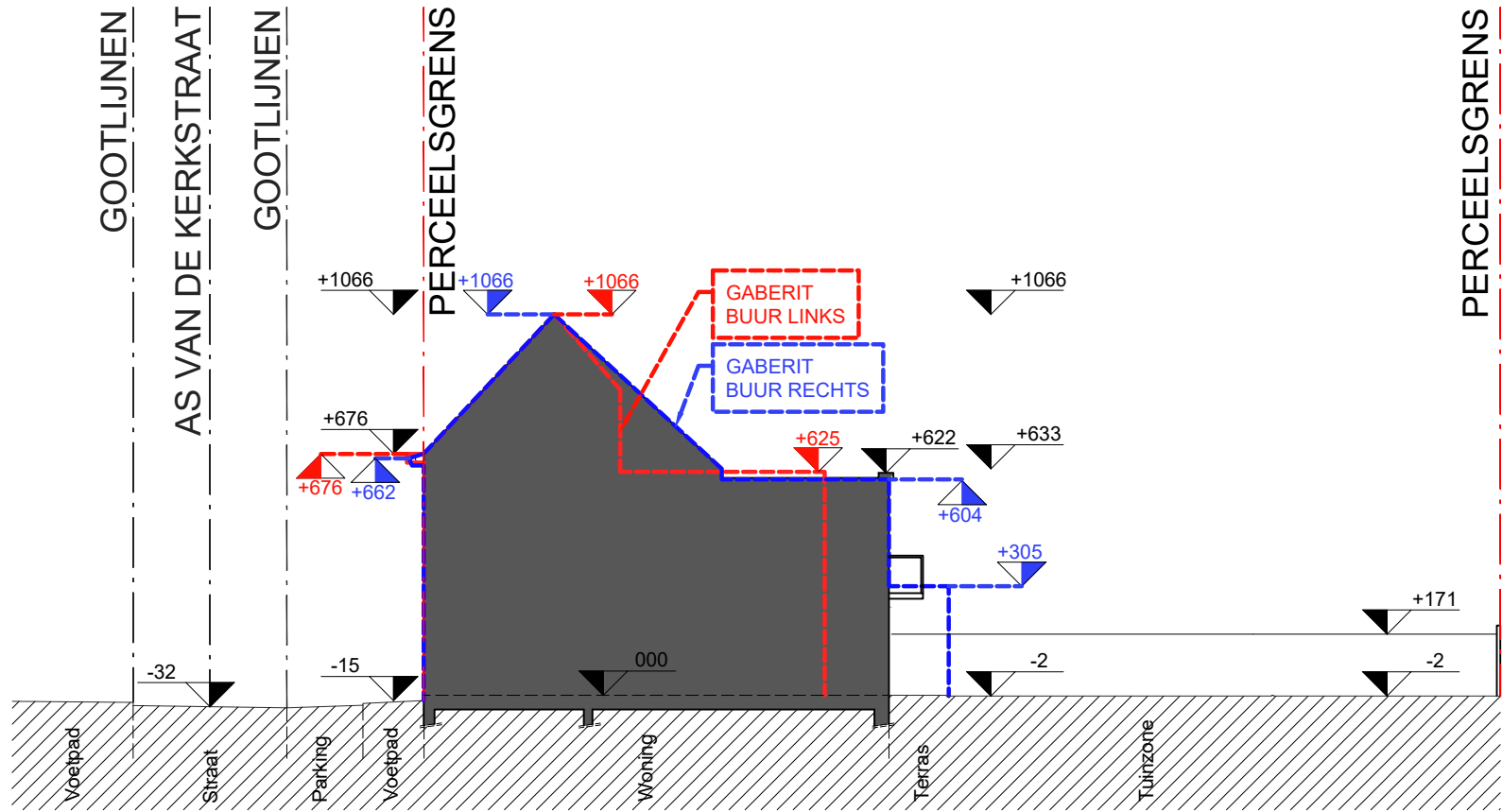
PLANNEN VERGUNDE TOESTAND: TERREINPROFIEL SCHAAL 1:200
