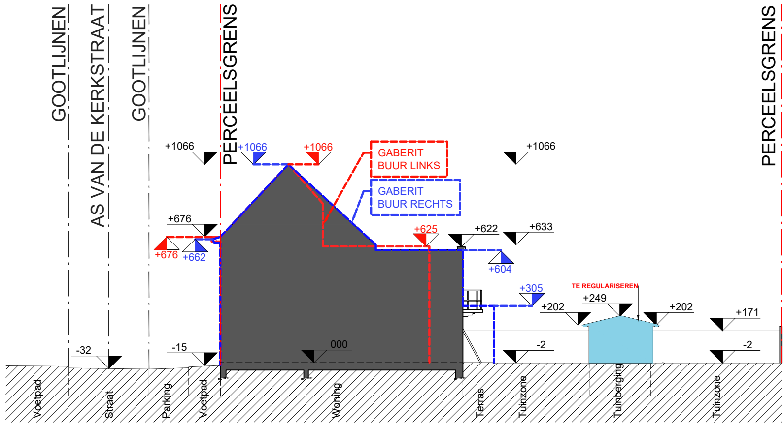
PLANNEN BESTAANDE TOESTAND: TERREINPROFIEL SCHAAL 1:200
