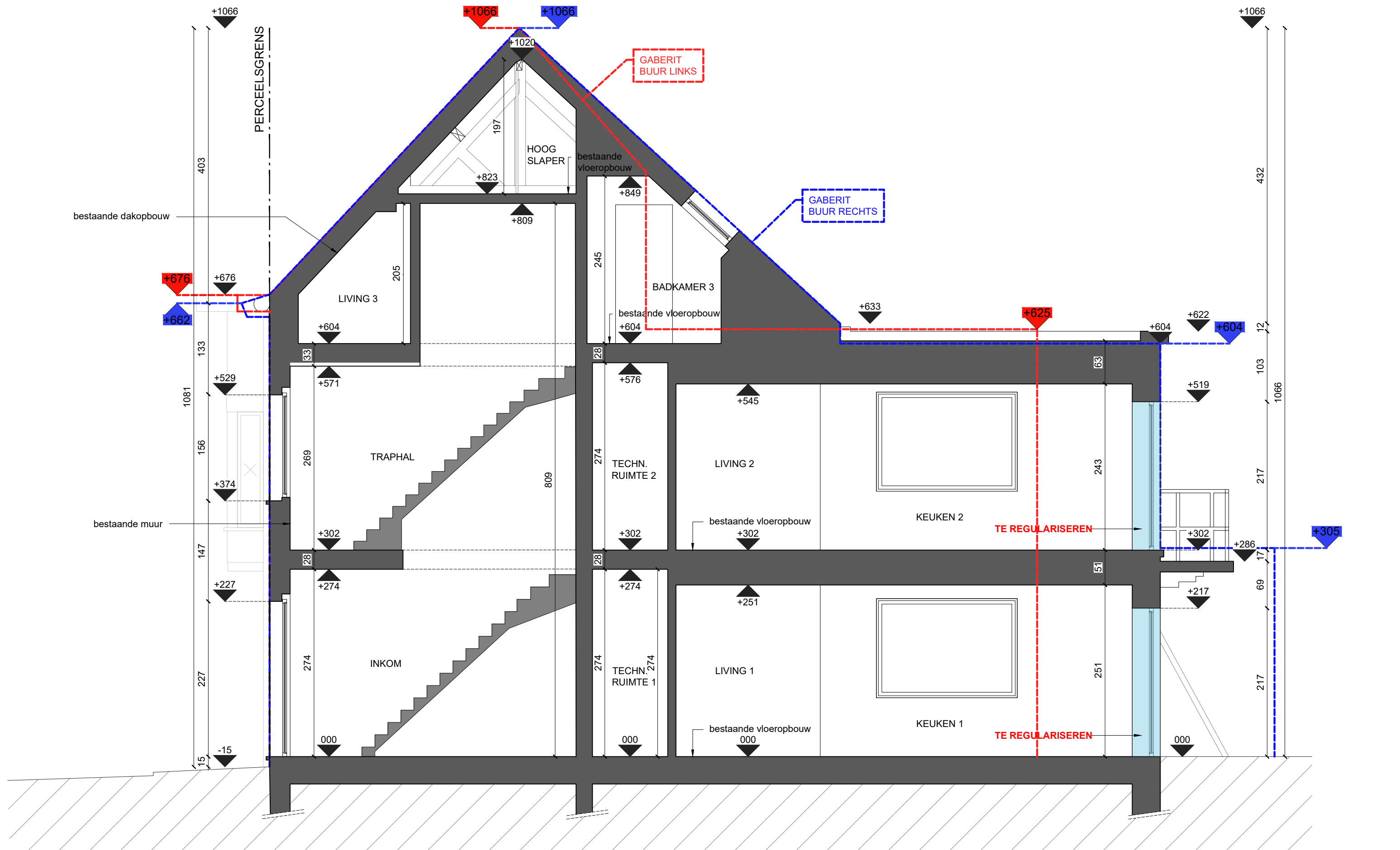
BESTAANDE TOESTAND: SNEDE A-A SCHAAL 1:50
