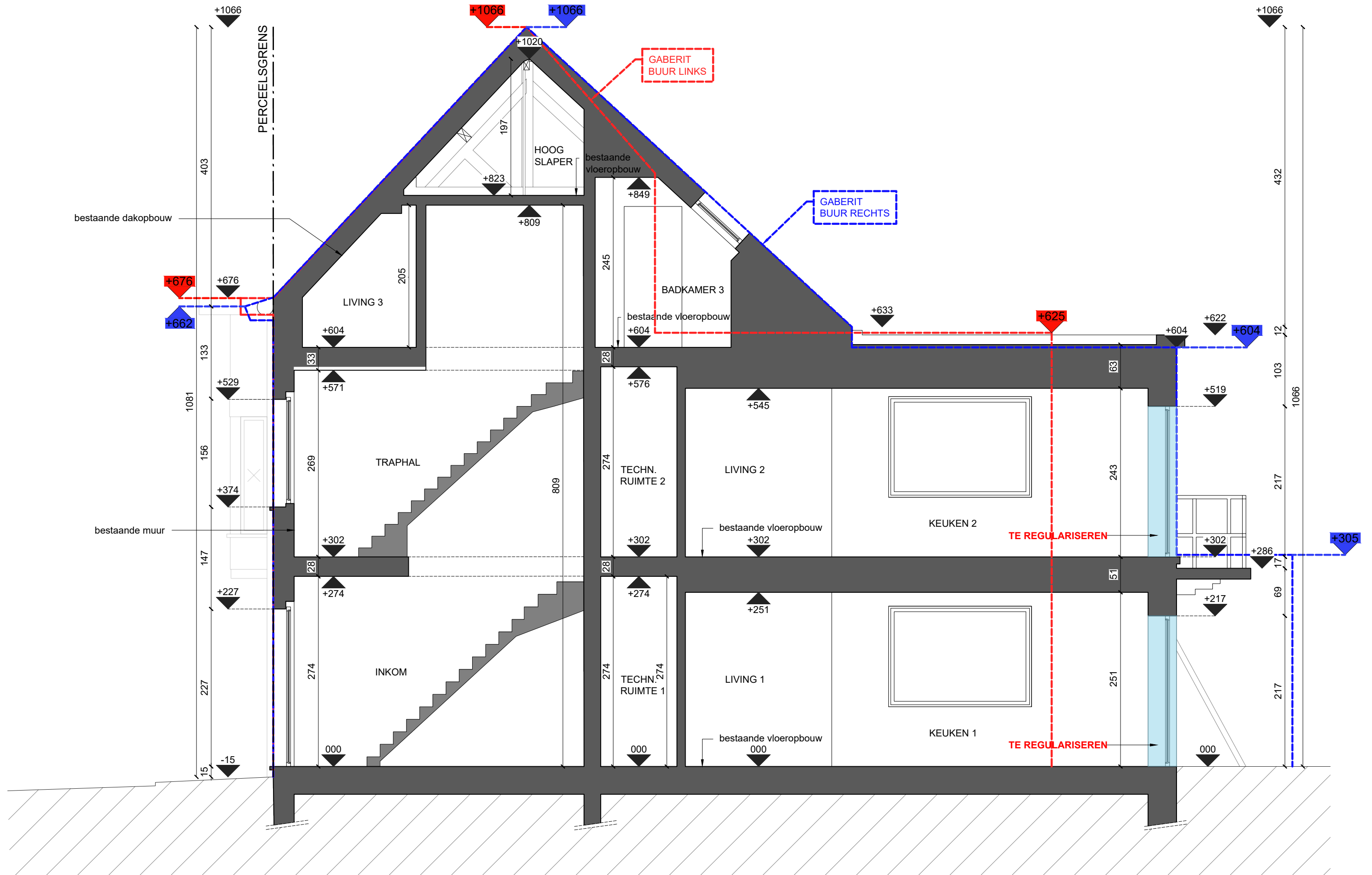
NIEUWE TOESTAND: SNEDE A-A SCHAAL 1:50
