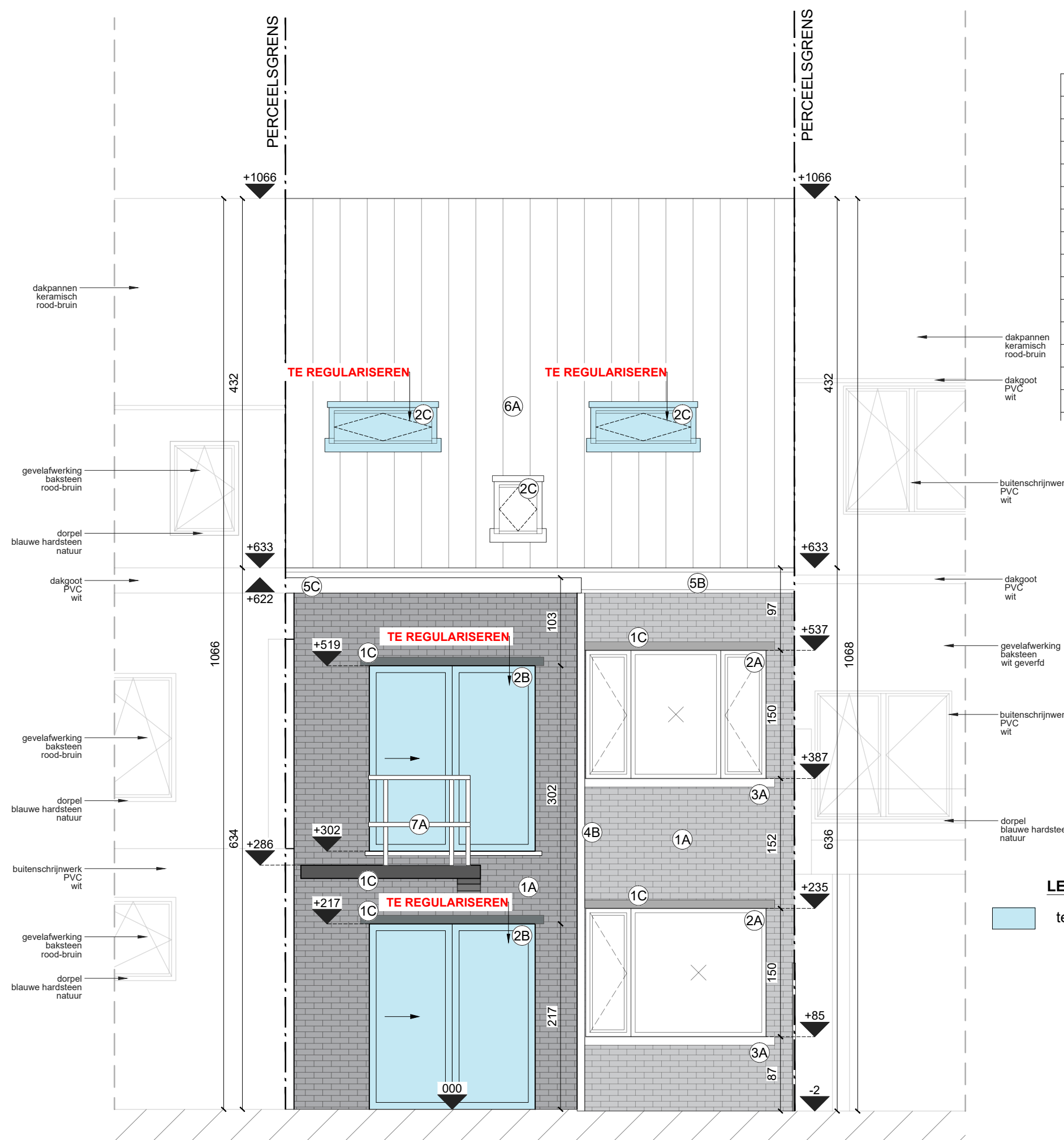
BESTAANDE TOESTAND: ACHTERGEVEL SCHAAL 1:50
