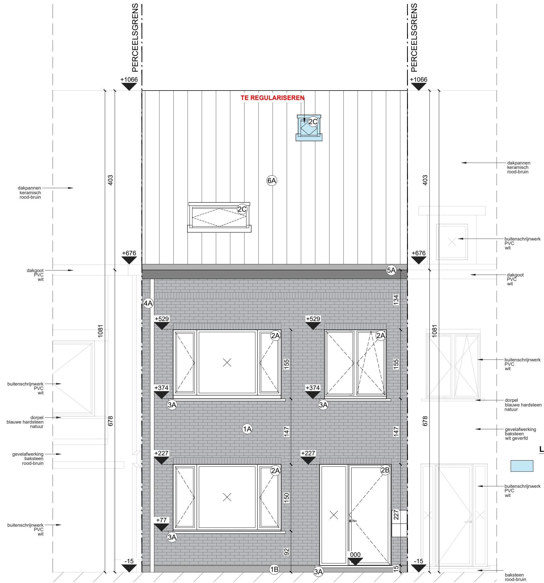
BESTAANDE TOESTAND: VOORGEVEL SCHAAL 1:50
