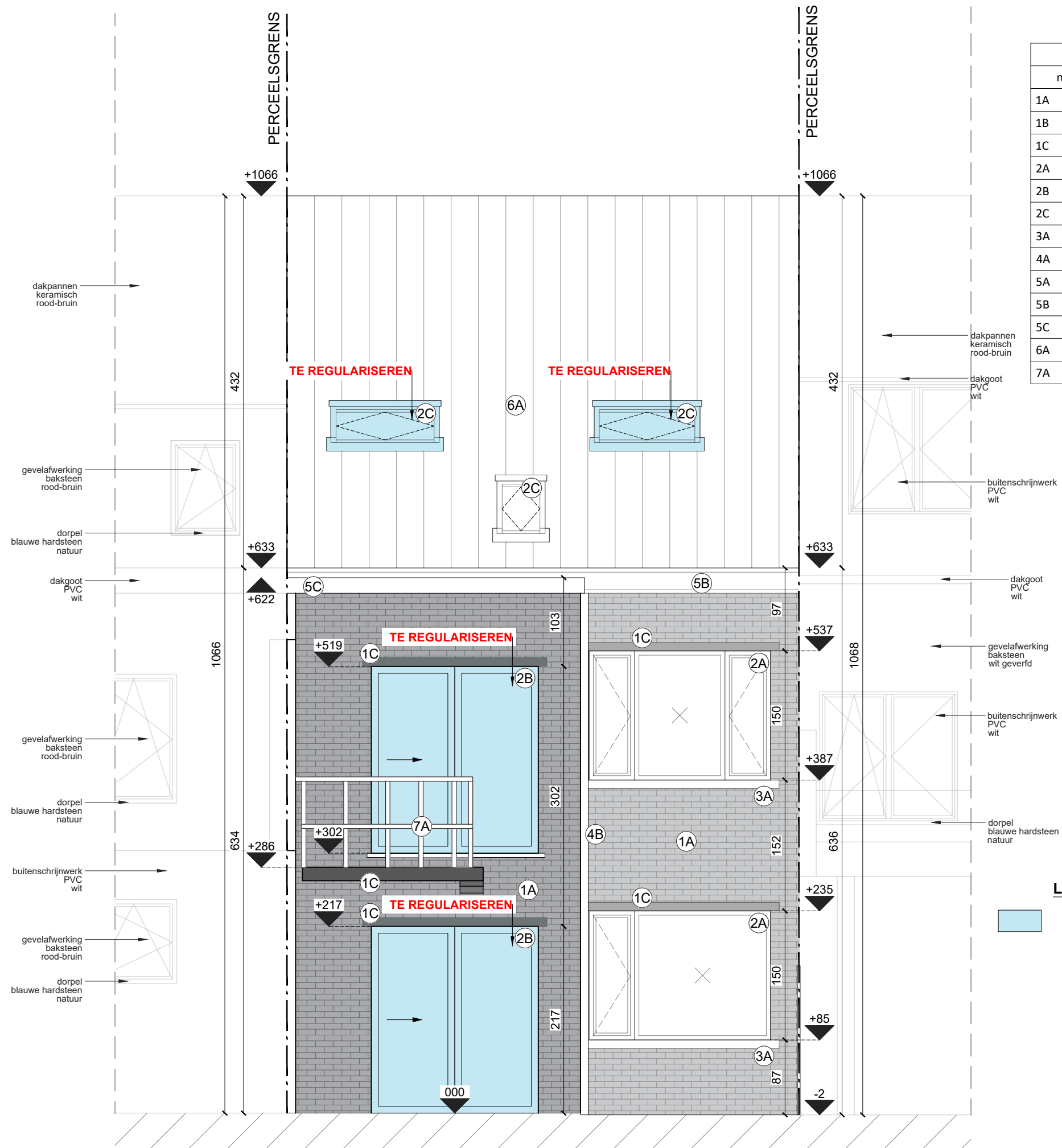
NIEUWE TOESTAND: ACHTERGEVEL SCHAAL 1:50
