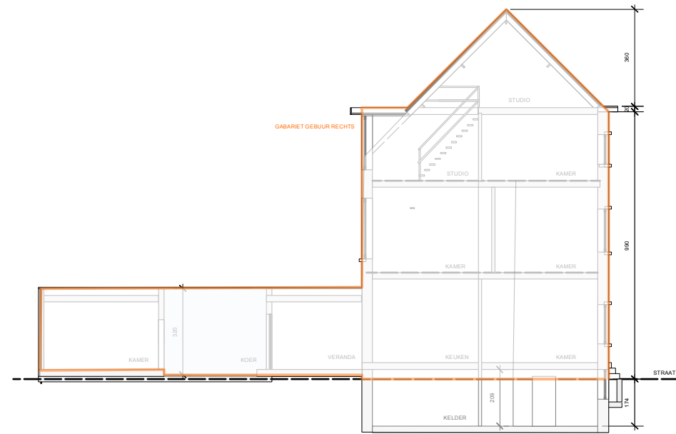
BA_REGULARISATIEAANVRAAG KAMERWONING_T_N_2_GABARIET GEBUUR RECHTS
