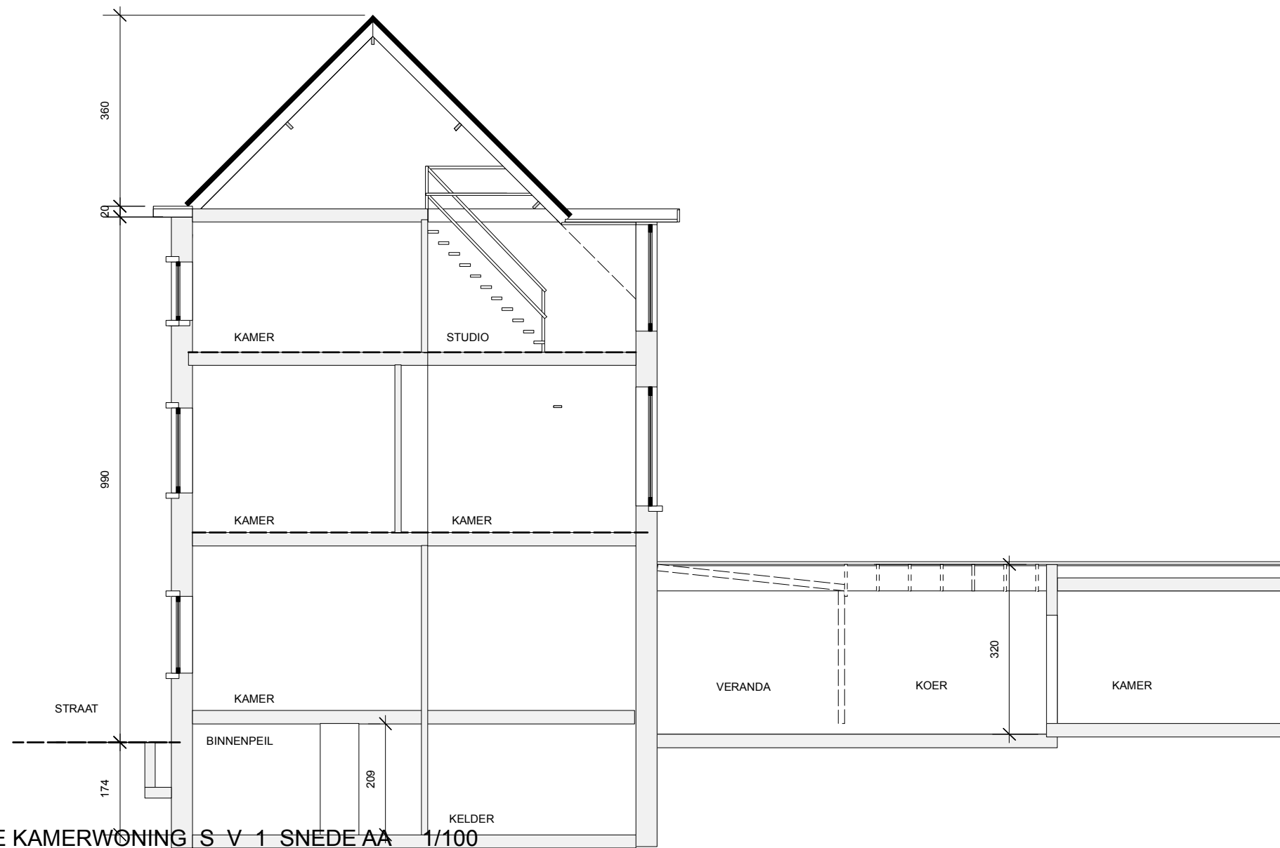
BA_REGULARISATIEAANVRAAG KAMERWONING_S_V_1_LANGSE SNEDE AA
