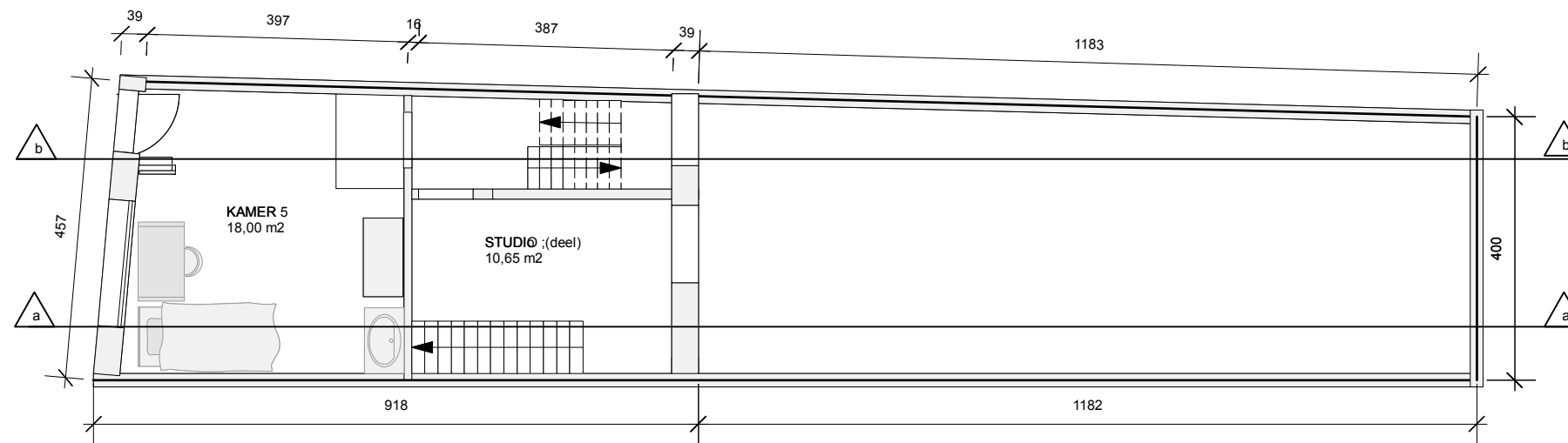
BA_REGULARISATIEAANVRAAG KAMERWONING_P_V_3 DAKVERDIEPING
