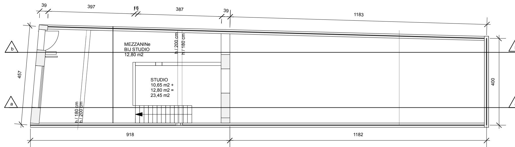
BA_REGULARISATIEAANVRAAG KAMERWONING_P_V_4_MEZZANINE
