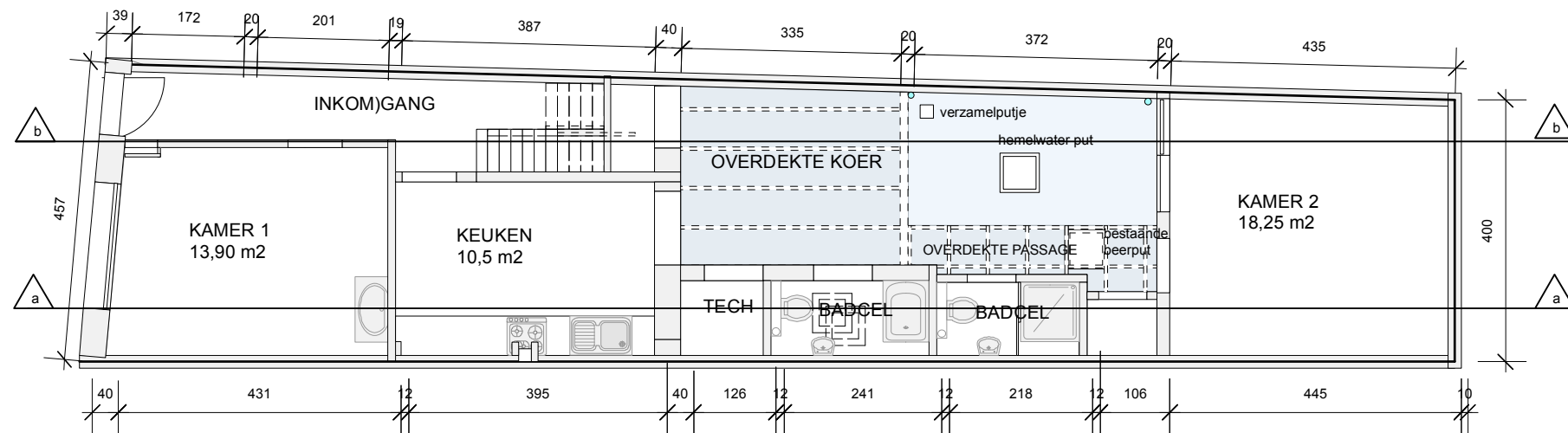
BA_REGULARISATIEAANVRAAG KAMERWONING_P_V_1_GELIJKVLOERS
