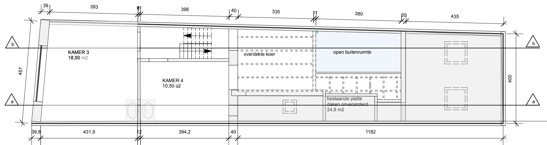
BA_REGULARISATIEAANVRAAG KAMERWONING_P_V_2_VERDIEPING
