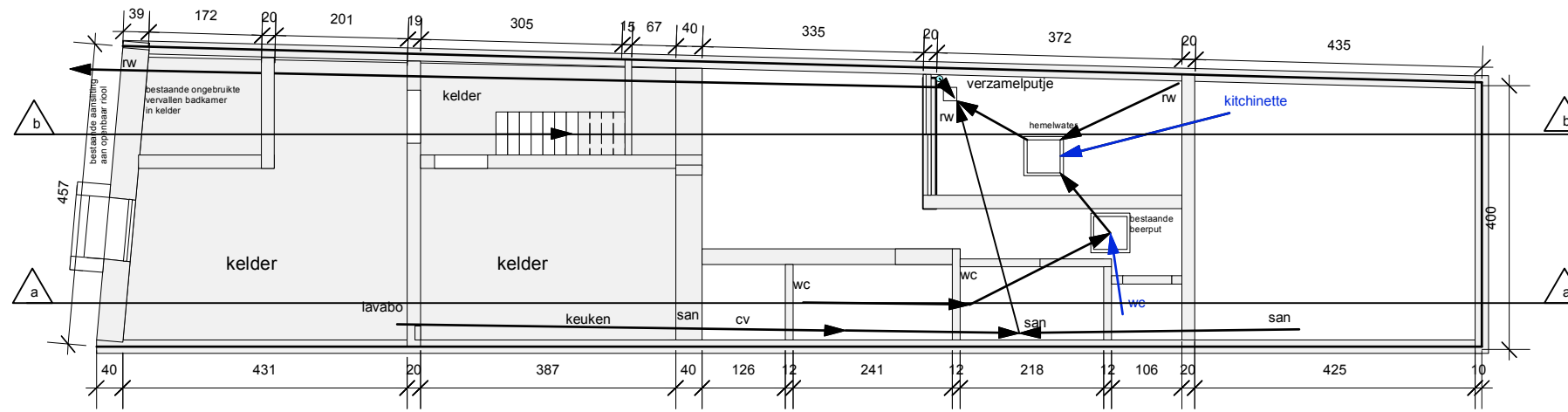
BA_REGULARISATIEAANVRAAG KAMERWONING_P_N_0_ONDERGROND
