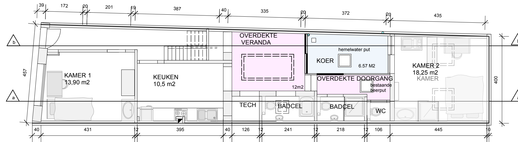
BA_REGULARISATIEAANVRAAG KAMERWONING_P_N_1_GELIJKVLOERS
