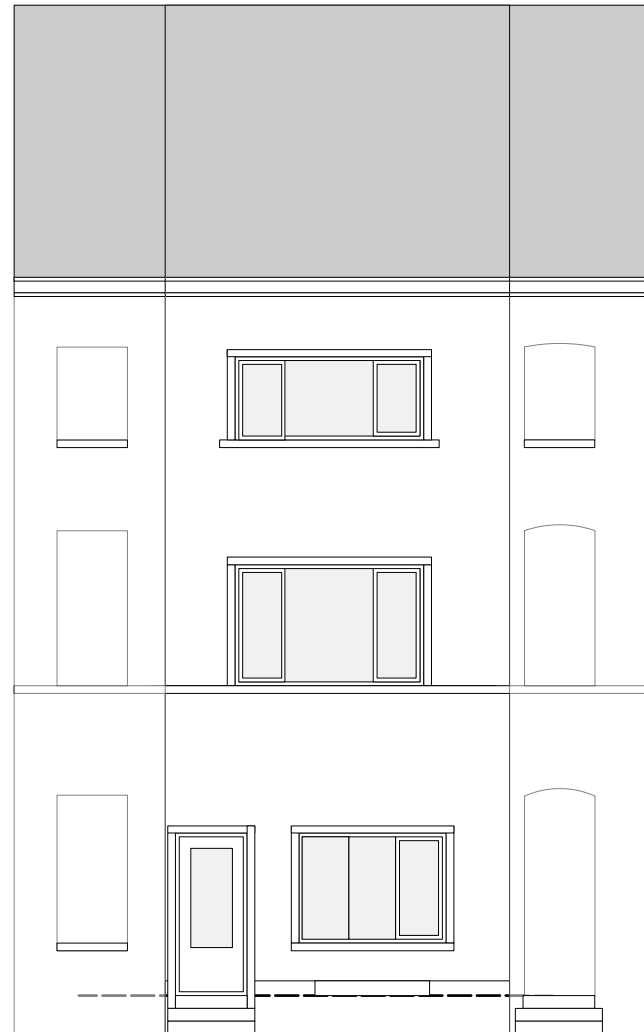
BA_REGULARISATIEAANVRAAG KAMERWONING_ G_N_1 STRAATGEVEL
