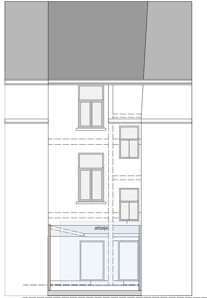
BA_REGULARISATIEAANVRAAG KAMERWONING_ 3_V_1_ACHTERGEVEL
