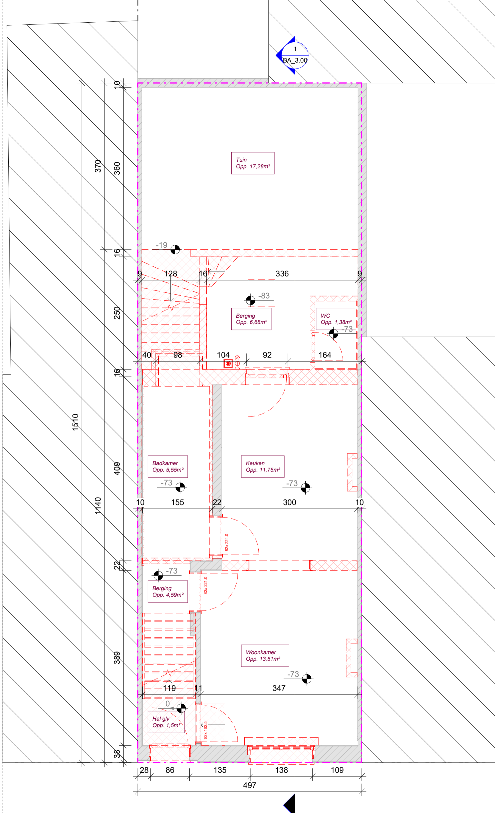
BA_1.00 P_B_1.00_Grondplan Gelijkvloers
