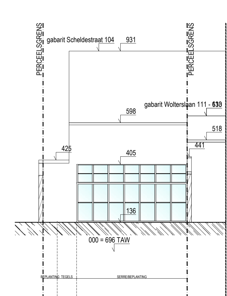
SNEDE DD'
