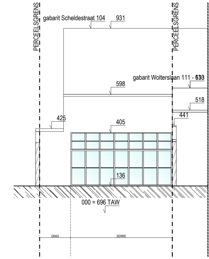
SNEDE DD'
