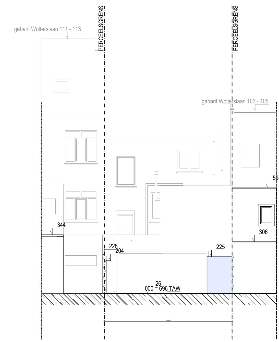
SNEDE CC'
