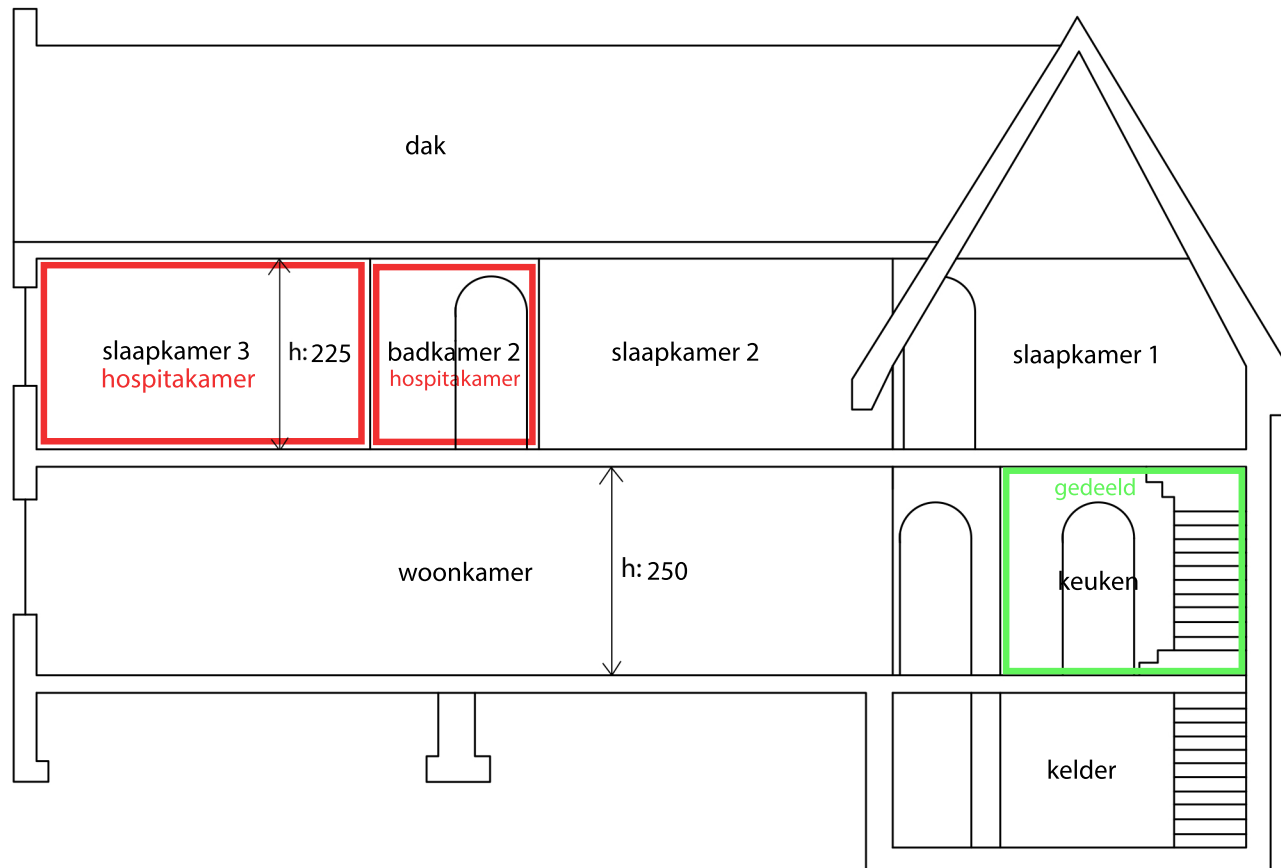
doorsnede nieuwe toestand schaal 1/100
