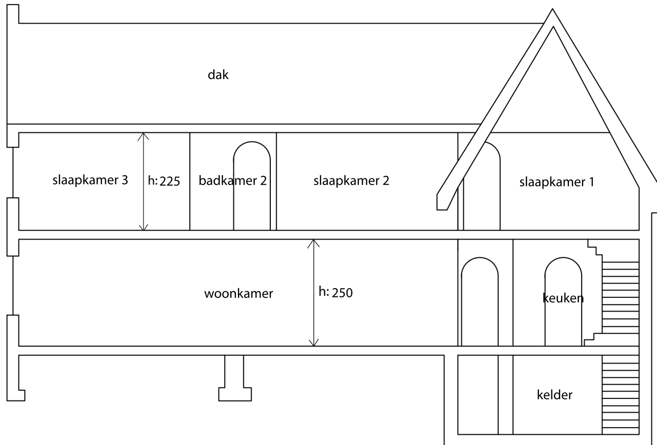
doorsnede bestaande toestand schaal 1/100
