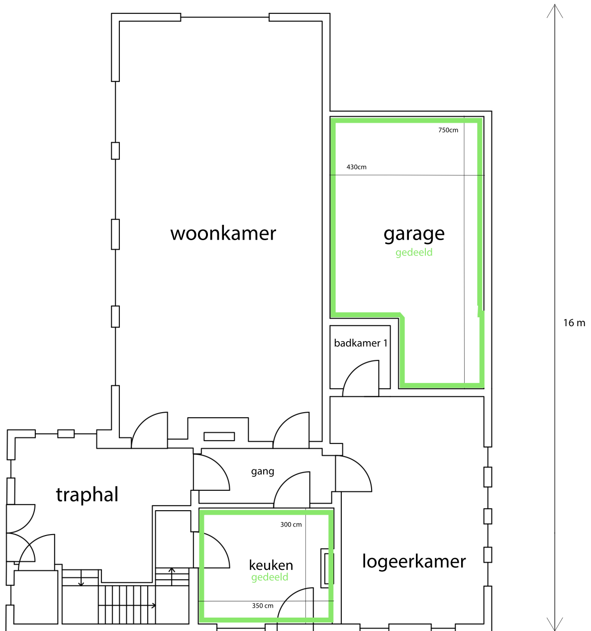
grondplan gelijkvloers nieuwe toestand schaal 1/100
