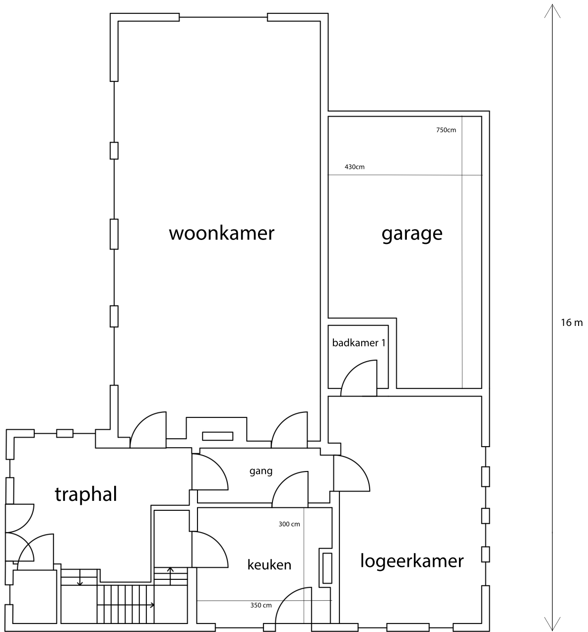
grondplan gelijkvloers bestaande toestand schaal 1/100
