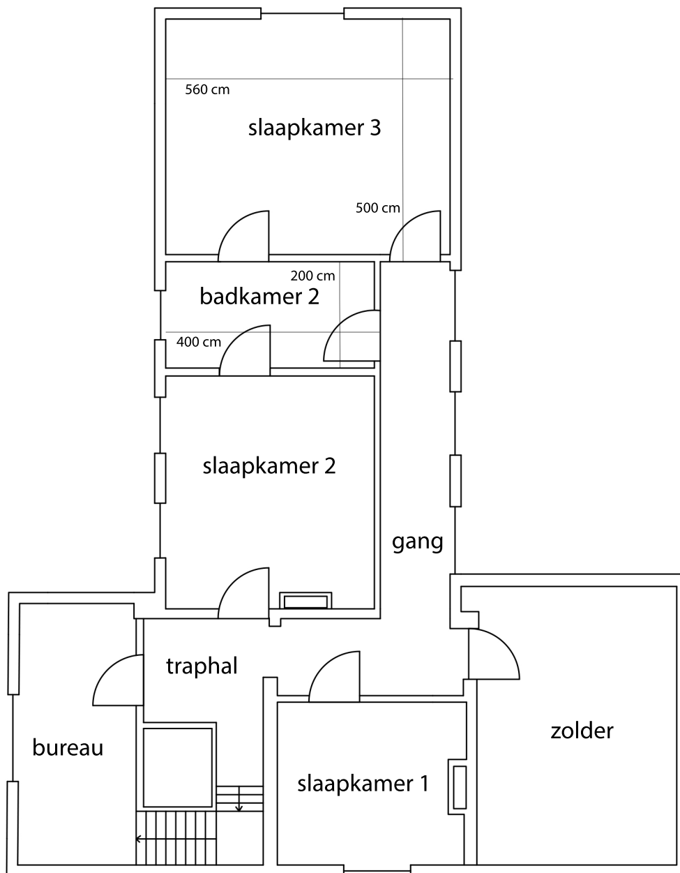
grondplan eerste verdieping bestaande toestand schaal 1/100
