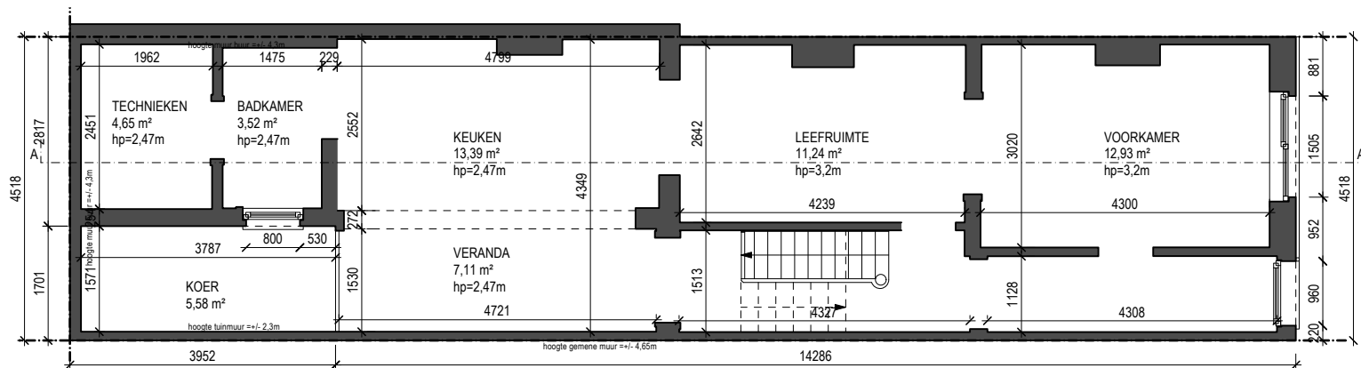
GELIJKVLOERS - 1/100 BESTAANDE TOESTAND
