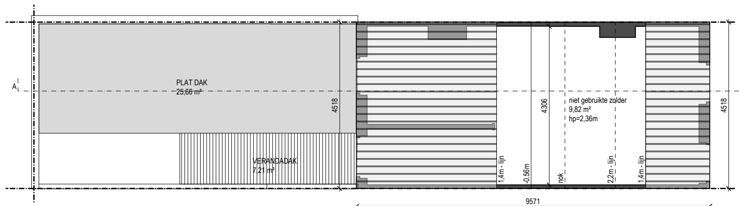
ZOLDER - 1/100 BESTAANDE TOESTAND
