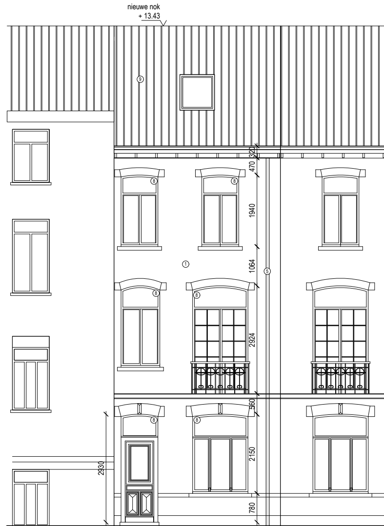
VOORGEVEL NIEUWE TOESTAND 1/100
