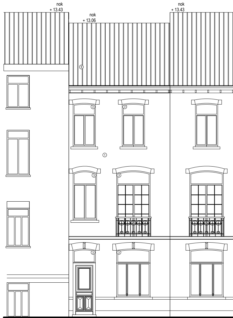
VOORGEVEL BESTAANDE TOESTAND 1/100
