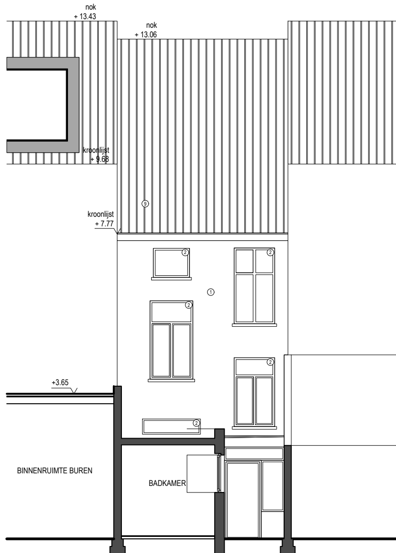
DWARSE SNEDE + ACHTERGEVEL BESTAANDE TOESTAND 1/100
