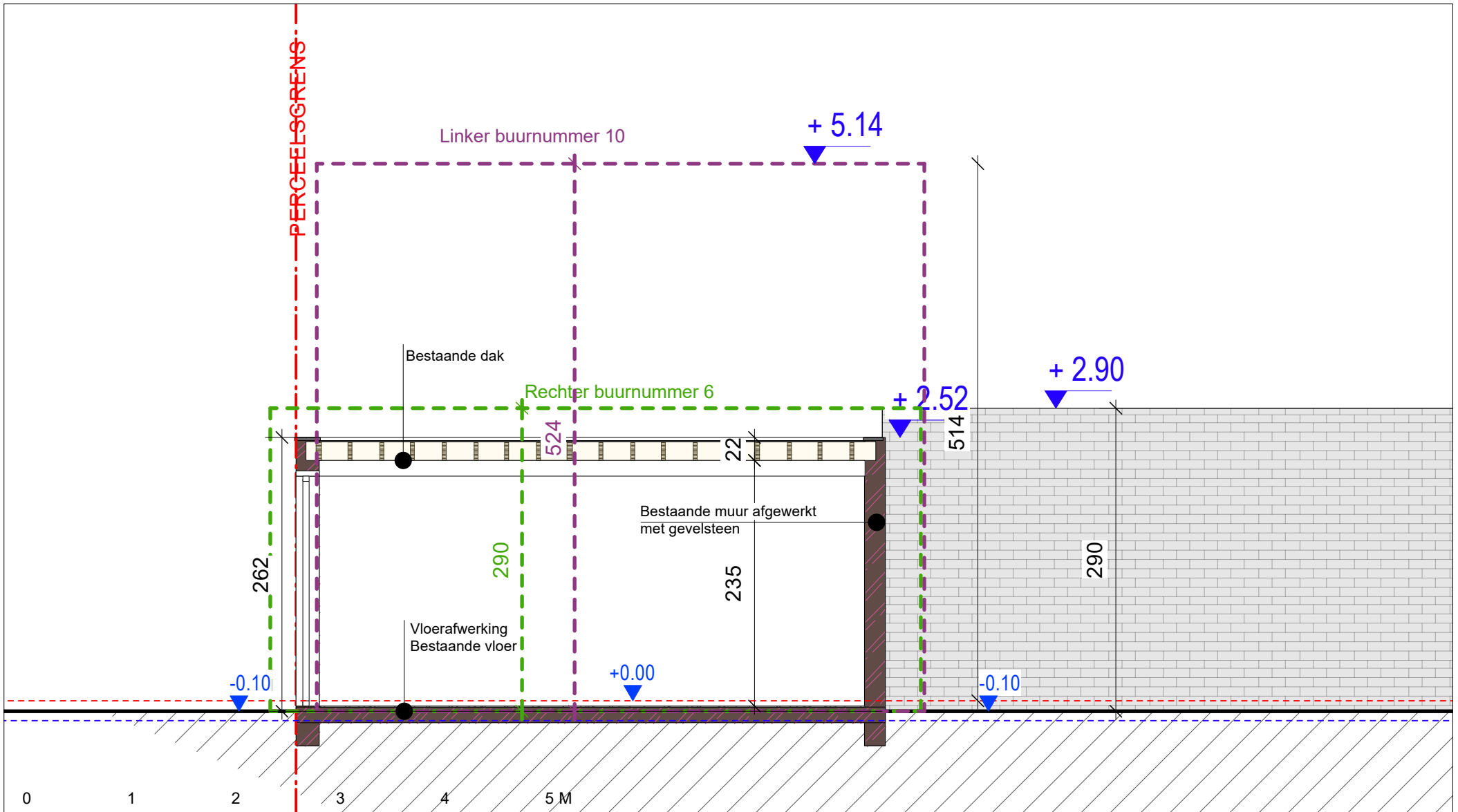
Garage Doorsnede VT Schaal: 1:50
