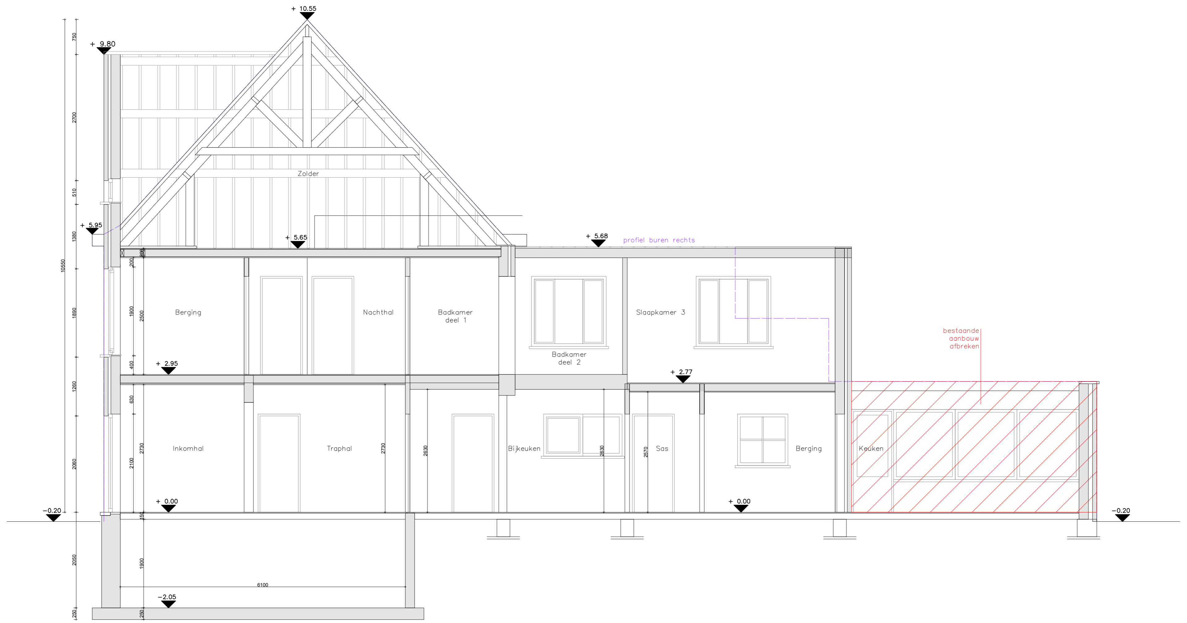
SNEDE A bestaande toestand schaal 1/50
