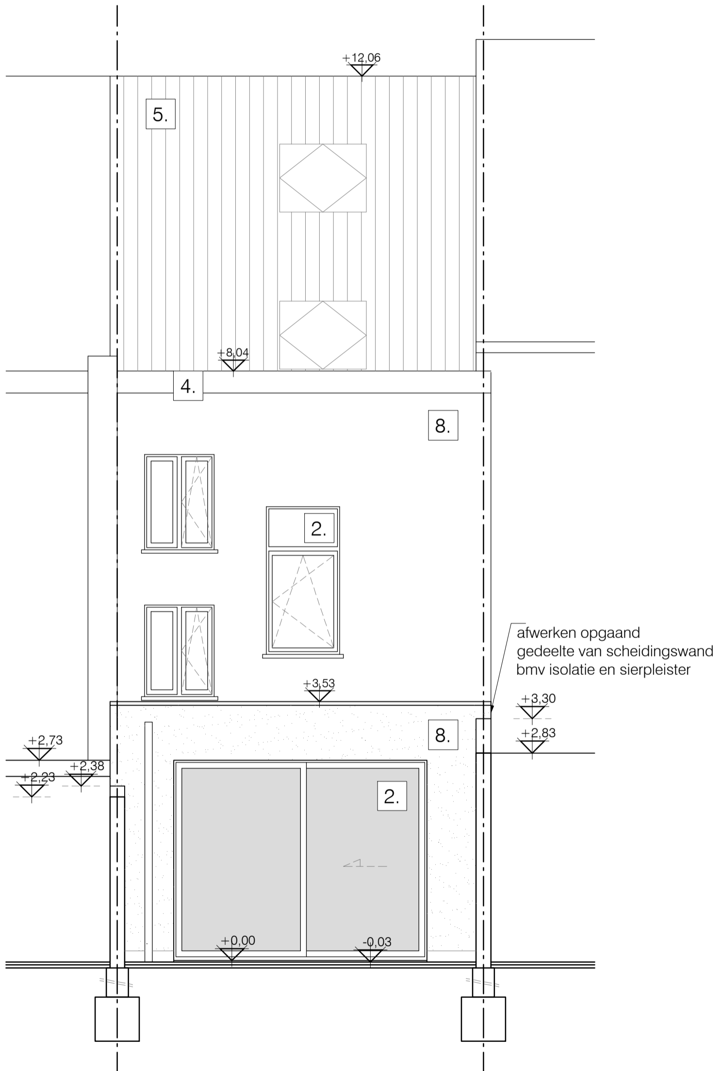
ACHTERGEVEL bestaande toestand alle afmetingen zijn in cm
