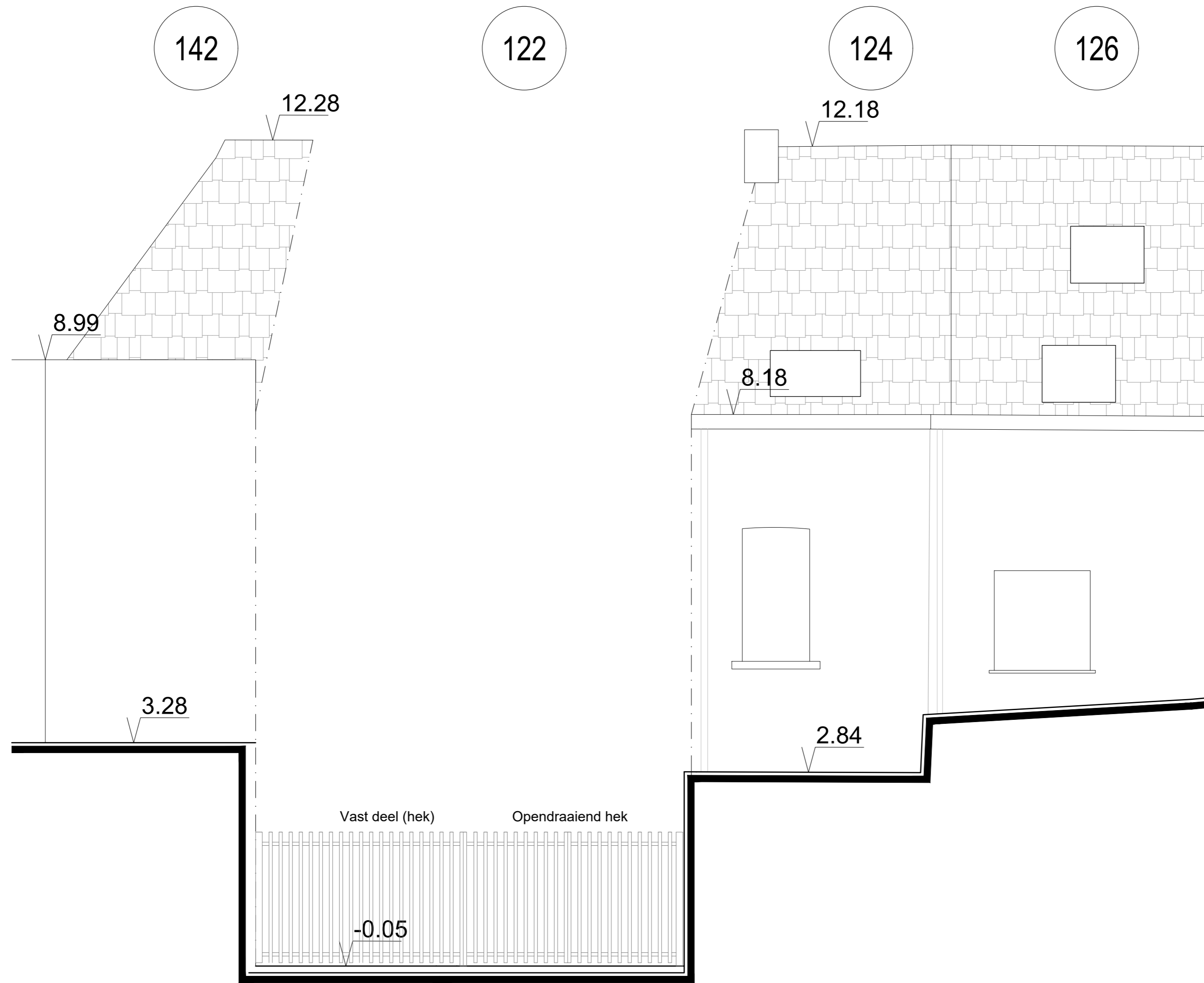
ACHTERGEVEL NIEUWE TOESTAND
