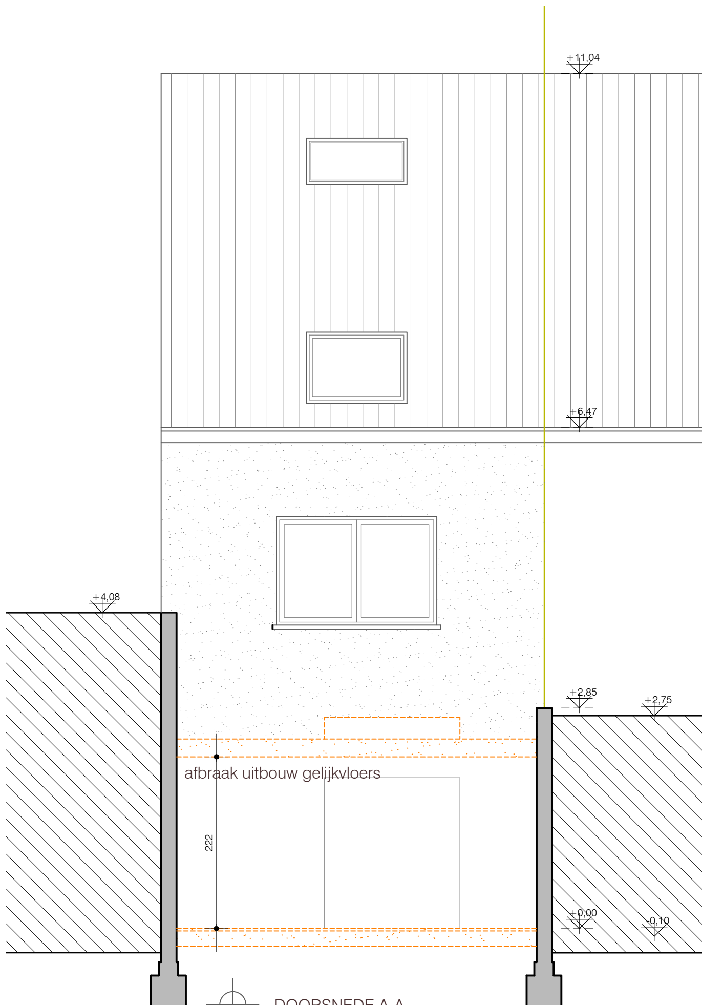
DOORSNEDE A-A schaal 1/50 afmetingen in cm bestaande toestand
