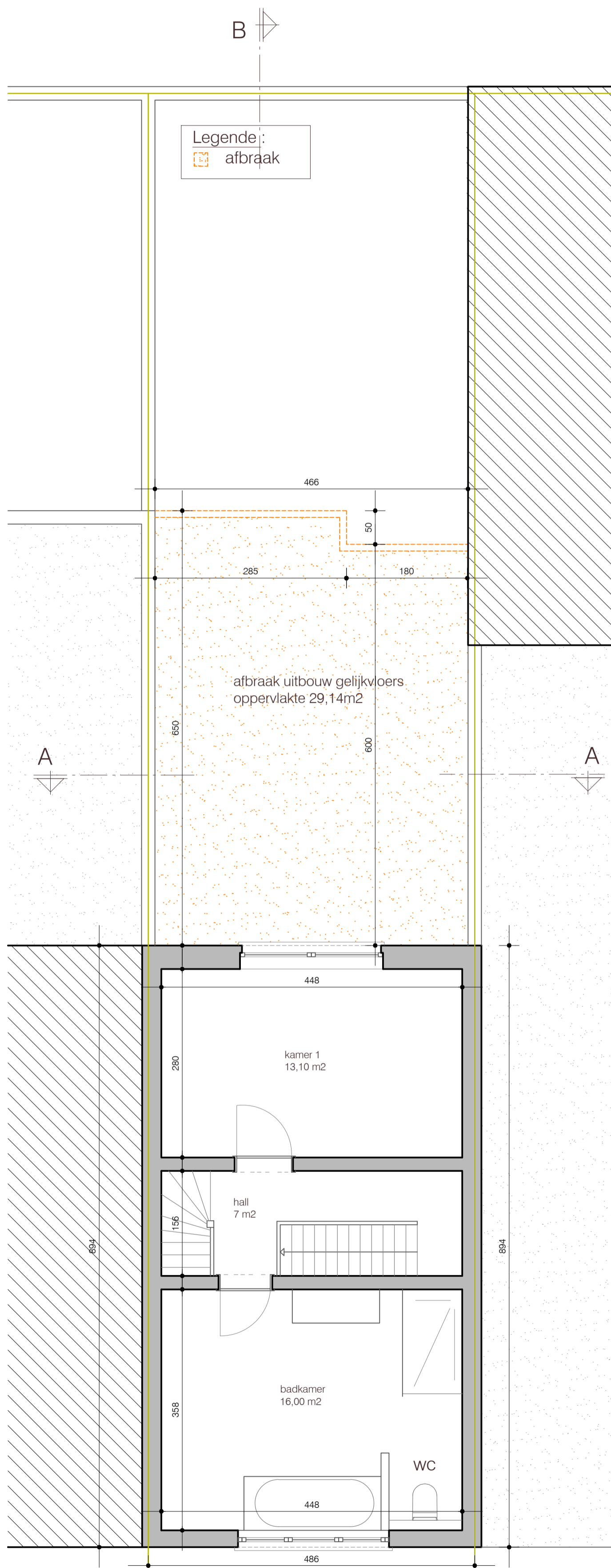
PLAN VERDIEPING +1 afmetingen in cm schaal 1/50 bestaande toestand
