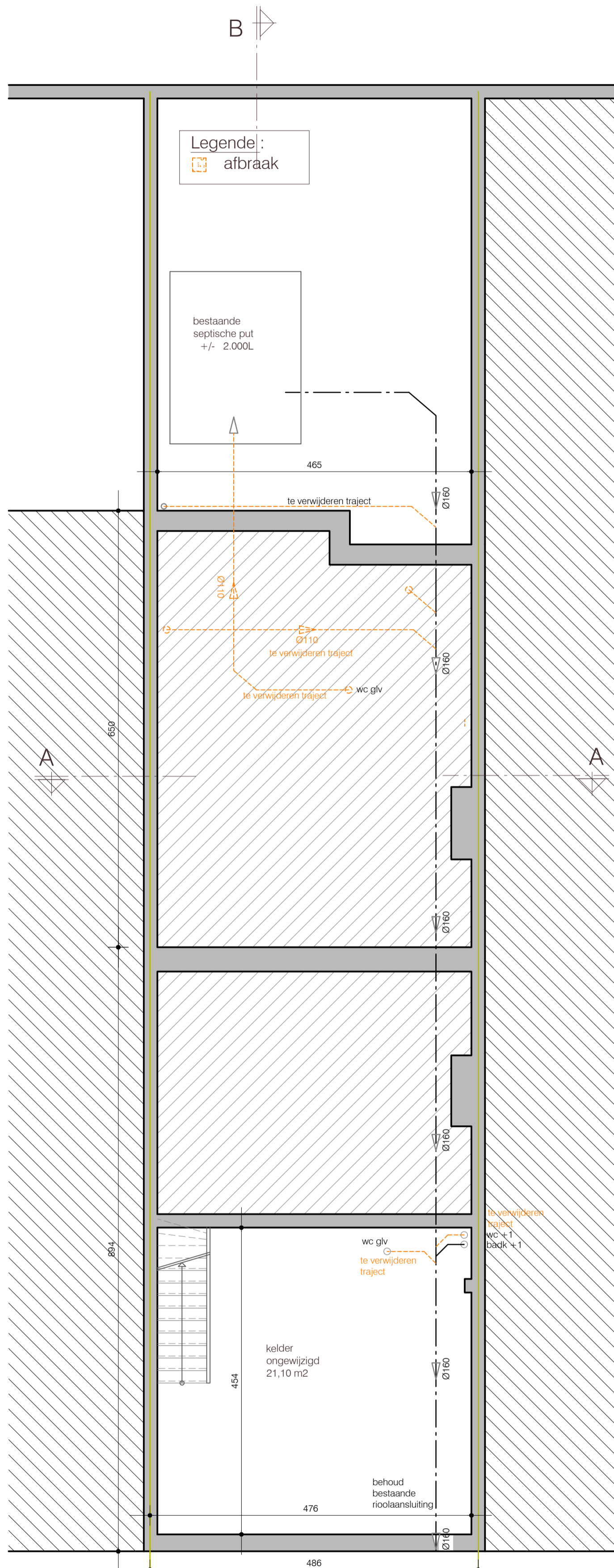
FUNDERING EN RIOLERINGSPLAN afmetingen in cm schaal 1/50 bestaande toestand
