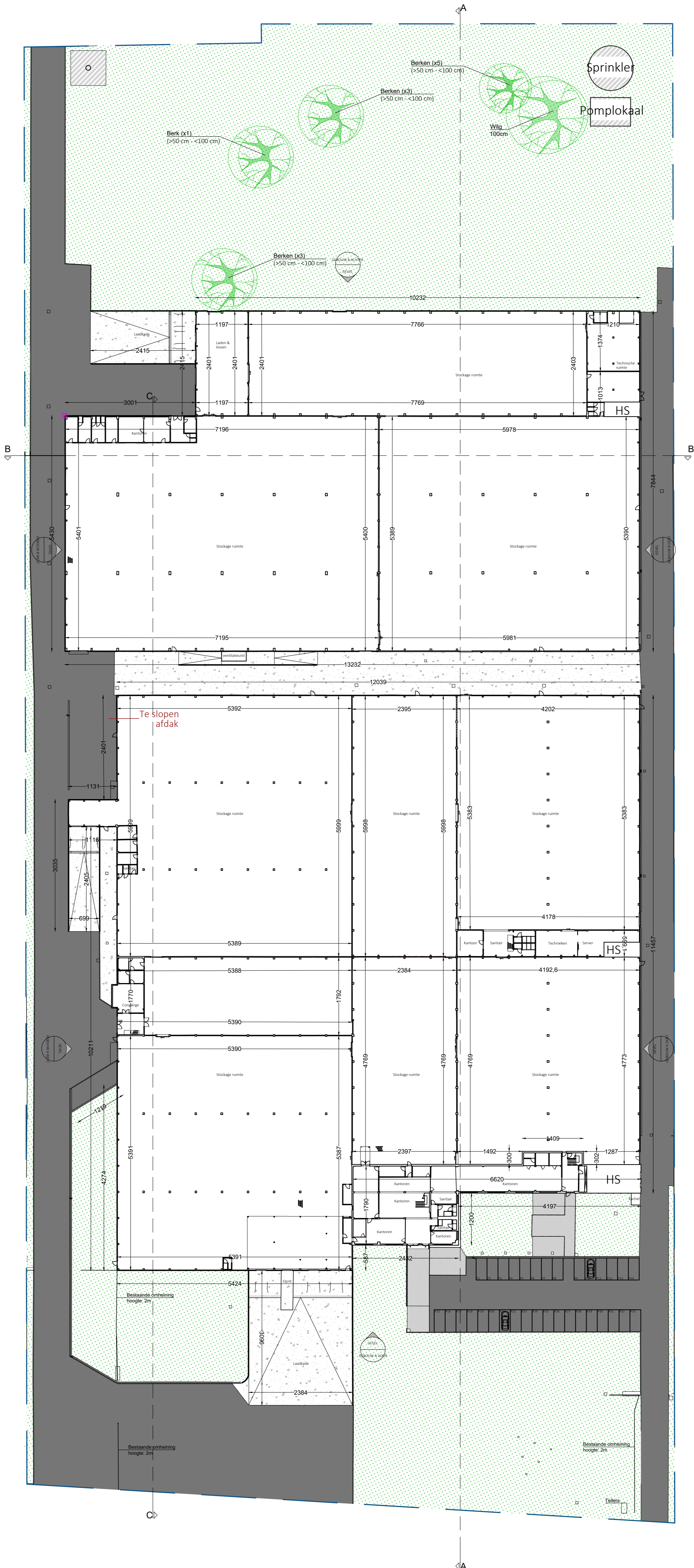
Overzichtplan gelijkvloers Vergunde toestand
