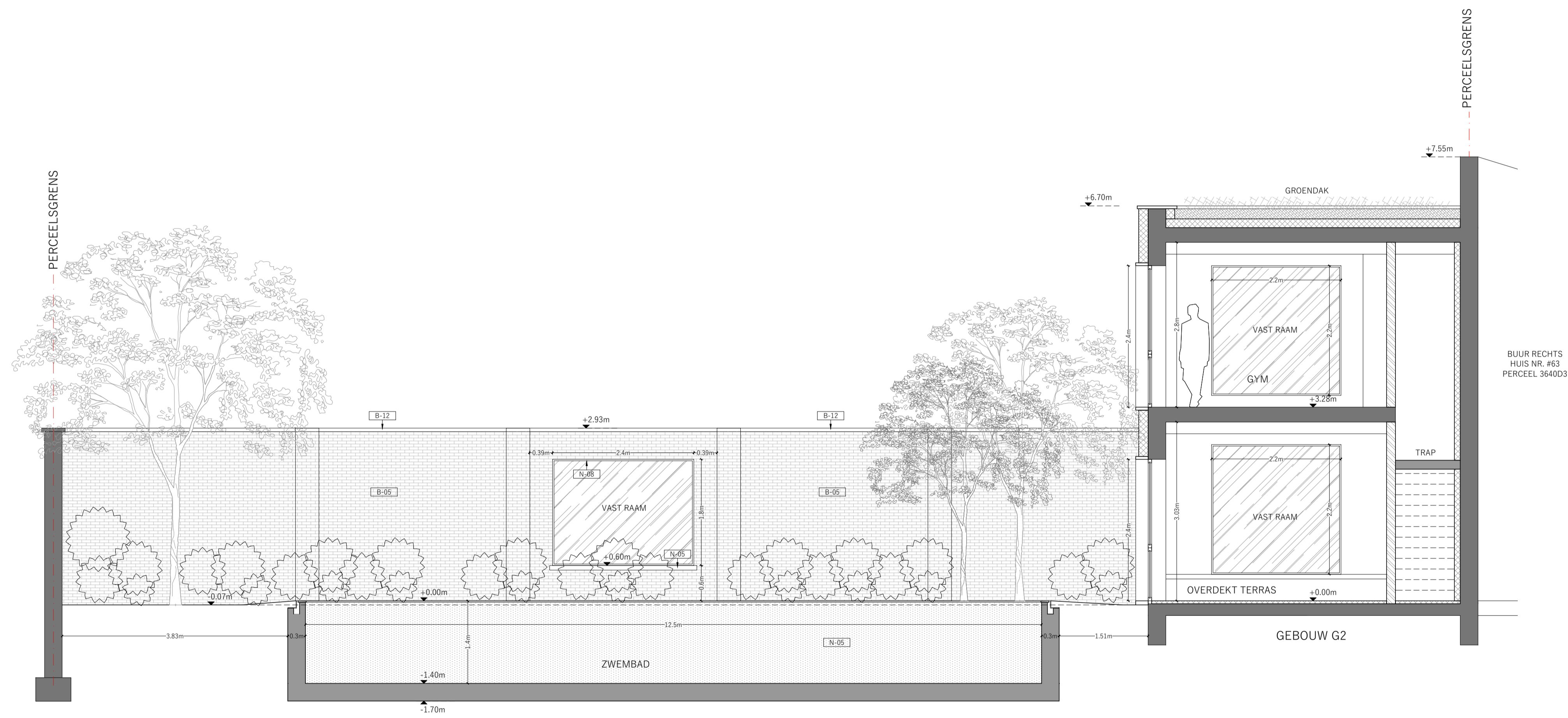
GEBOUW G2 | NIEUWE TOESTAND | SNEDE C | SCHAAL 1:50
