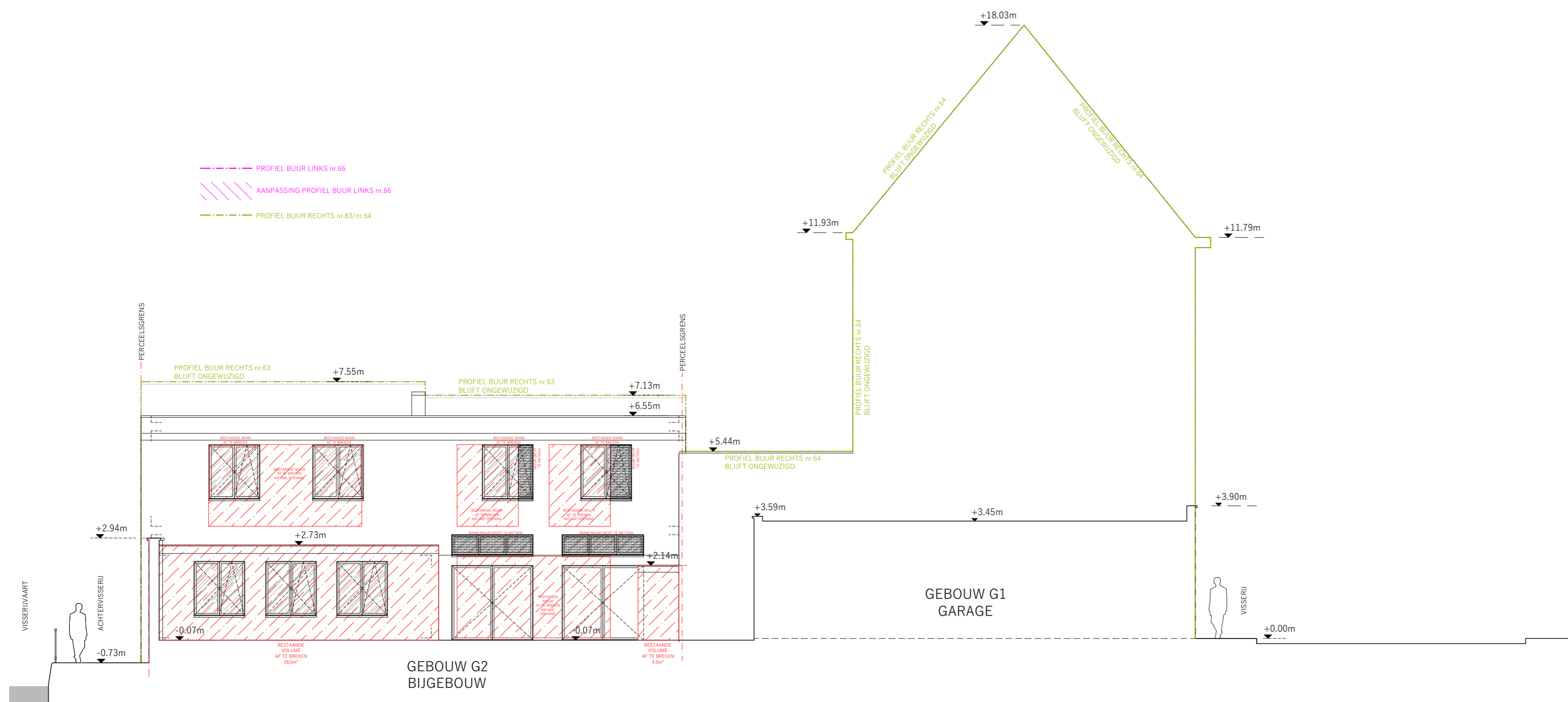
TERREIN PROFIEL C | BESTAANDE TOESTAND | SCHAAL 1:100
