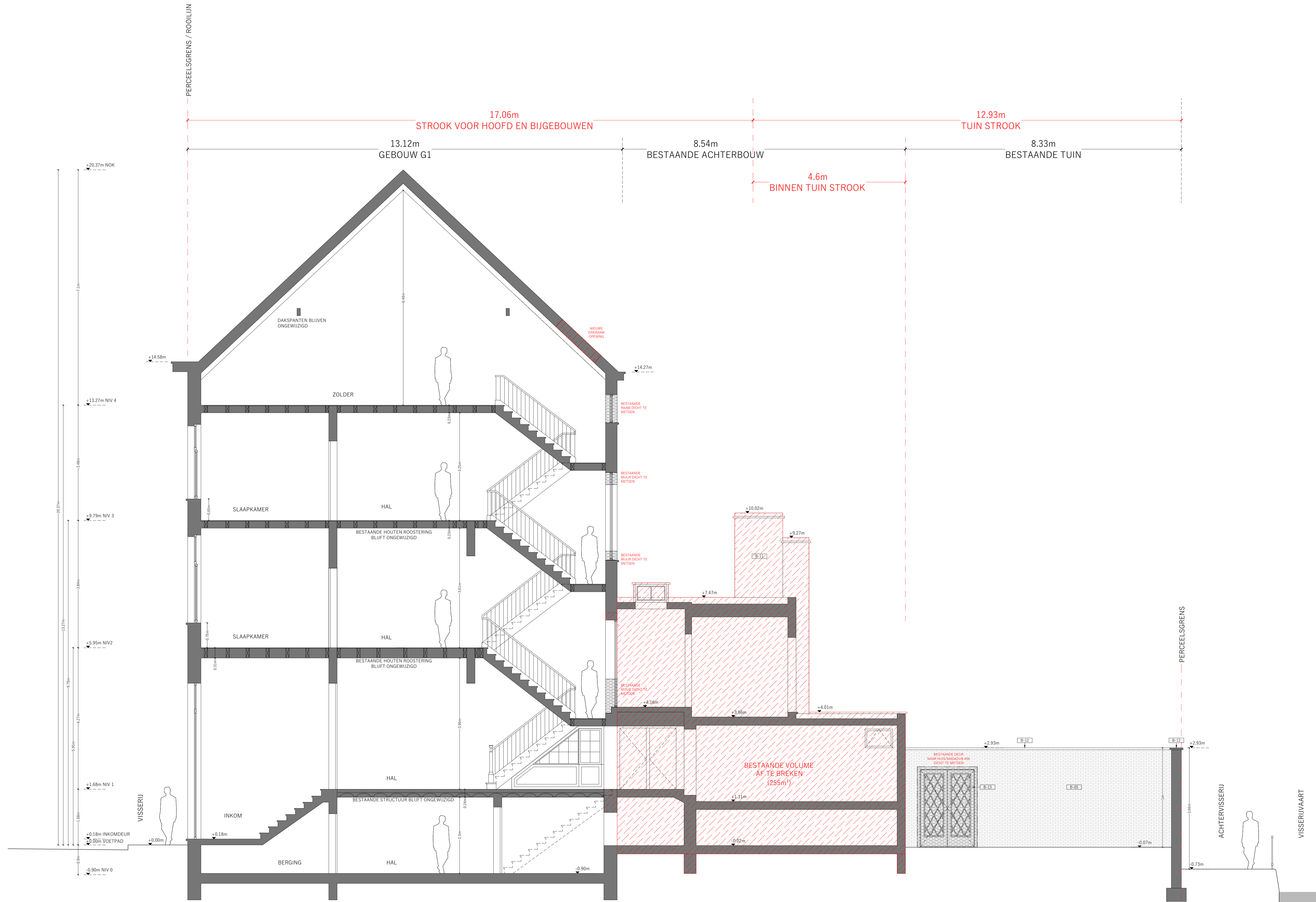
GEBOUW G1 | BESTAANDE TOESTAND | SNEDE B | SCHAAL 1:50
