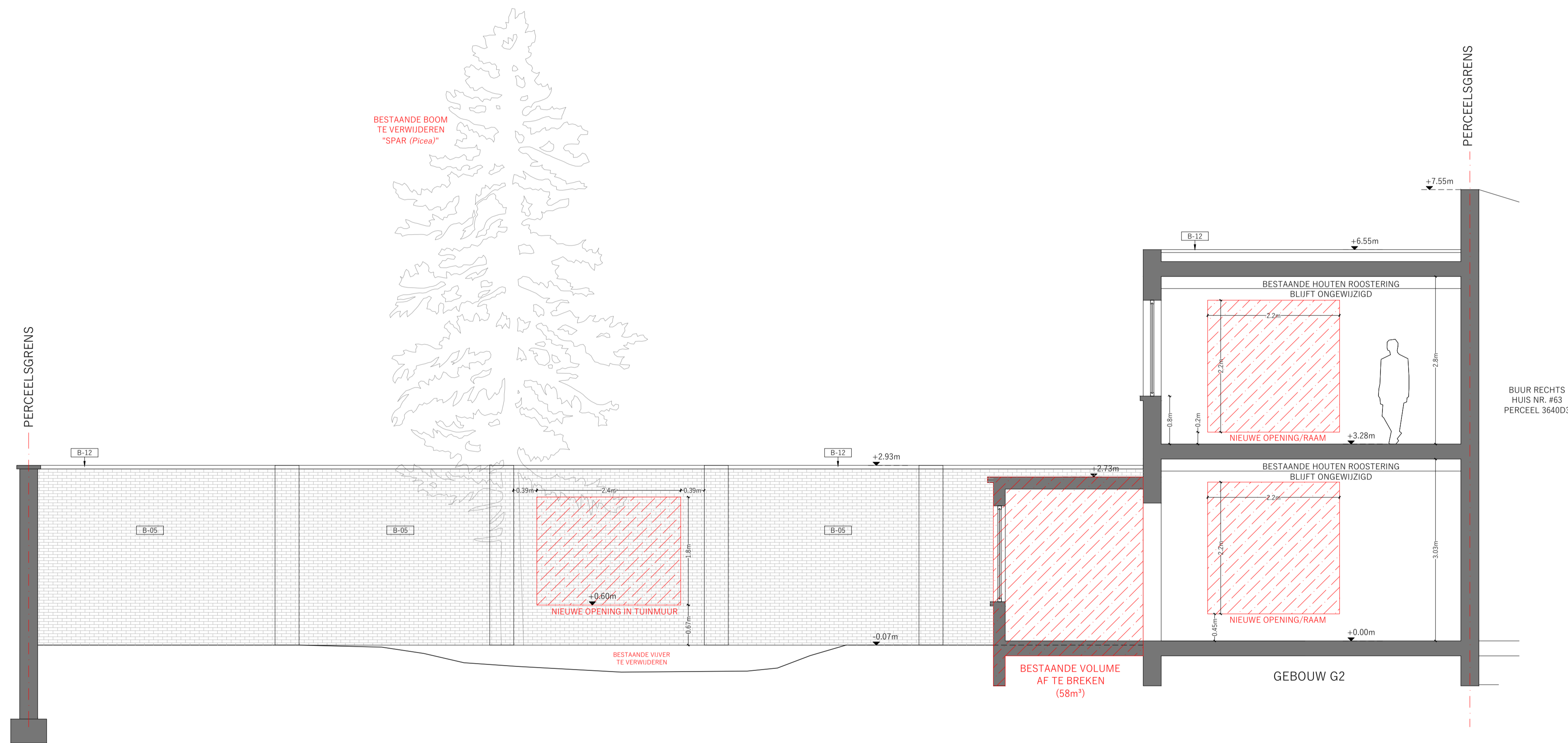
GEBOUW G2 | BESTAANDE TOESTAND | SNEDE C | SCHAAL 1:50
