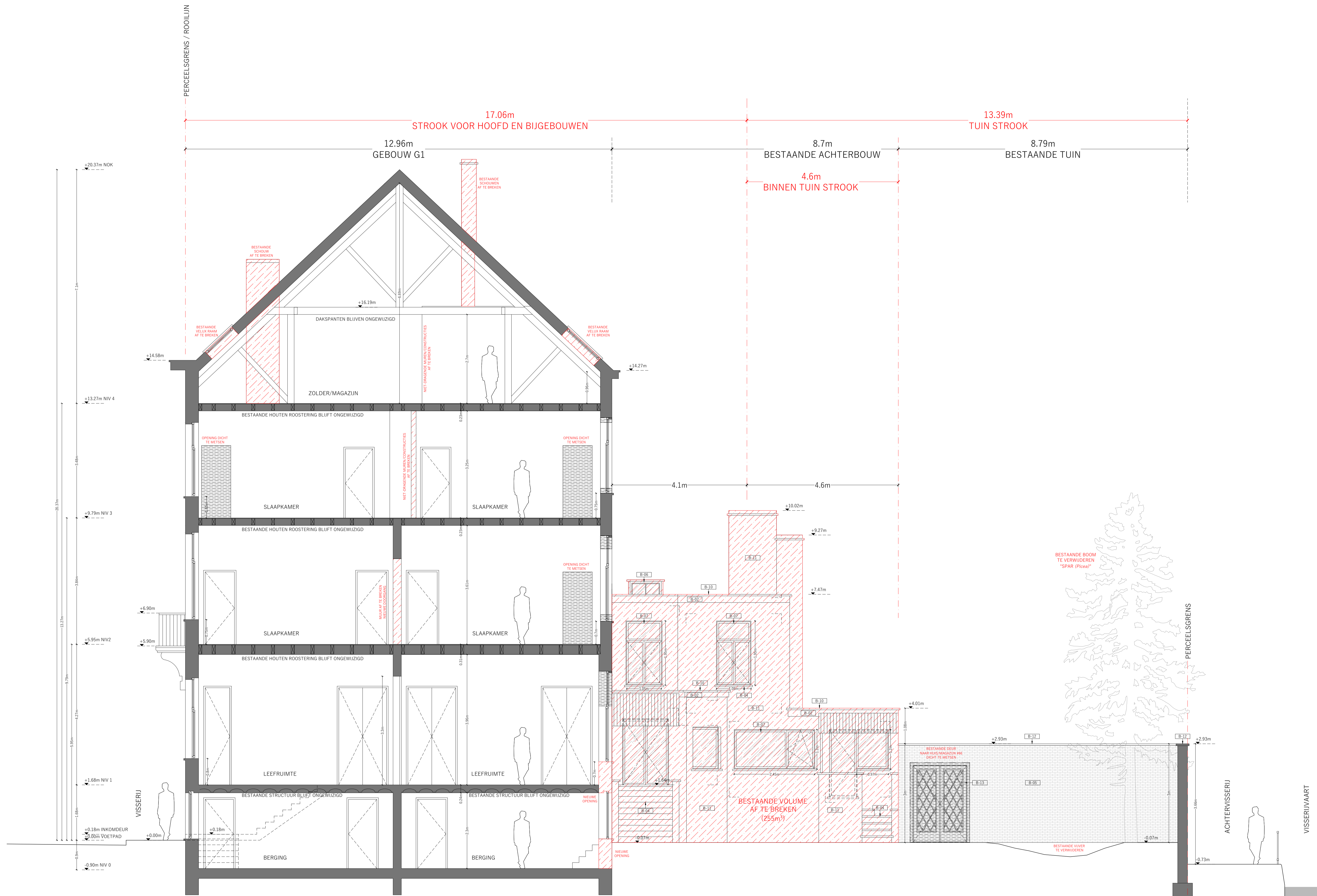
GEBOUW G1 | BESTAANDE TOESTAND | SNEDE A | SCHAAL 1:50
