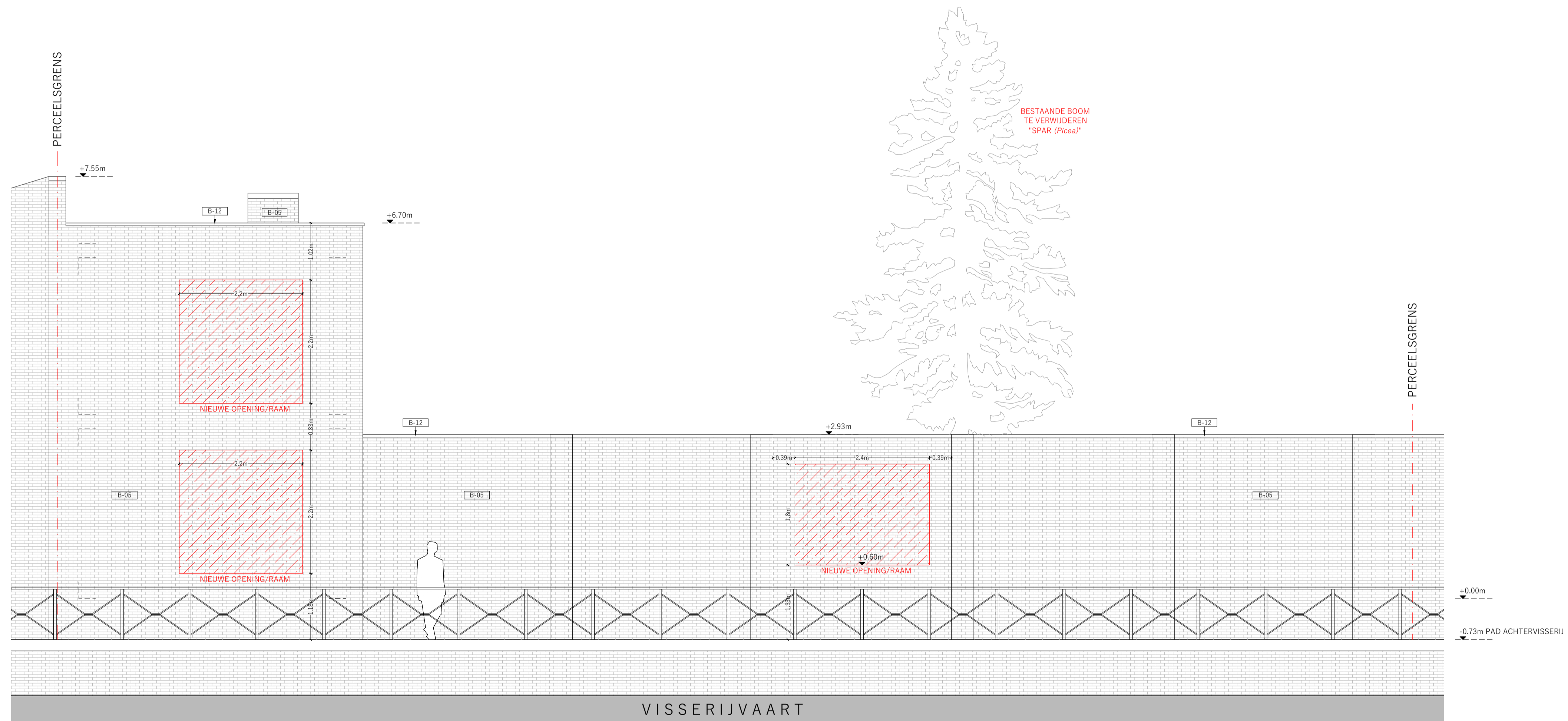
GEBOUW G2 | BESTAANDE TOESTAND | ACHTERGEVEL | SCHAAL 1:50
