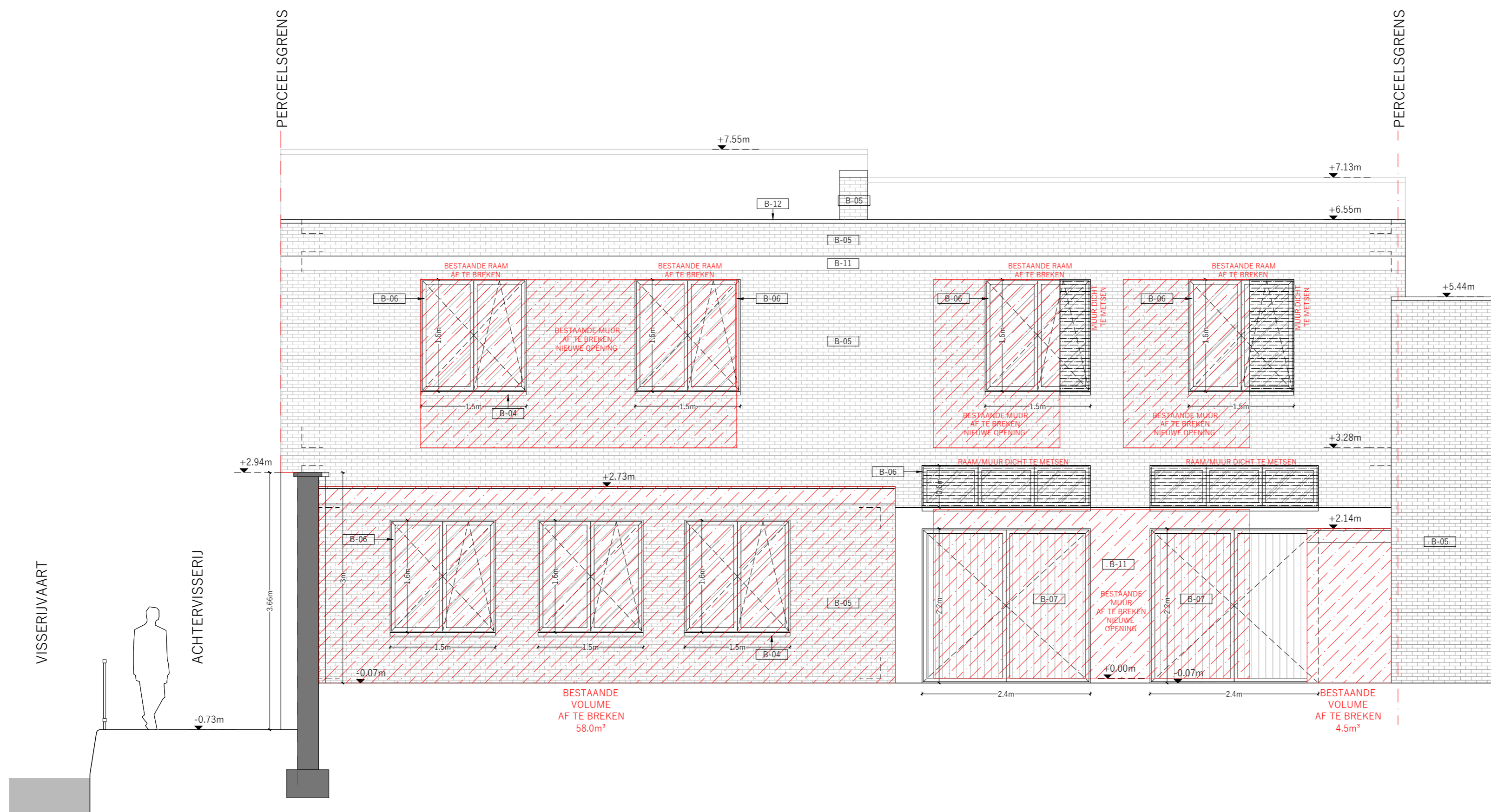
GEBOUW G2 | BESTAANDE TOESTAND | VOORGEVEL | SCHAAL 1:50
