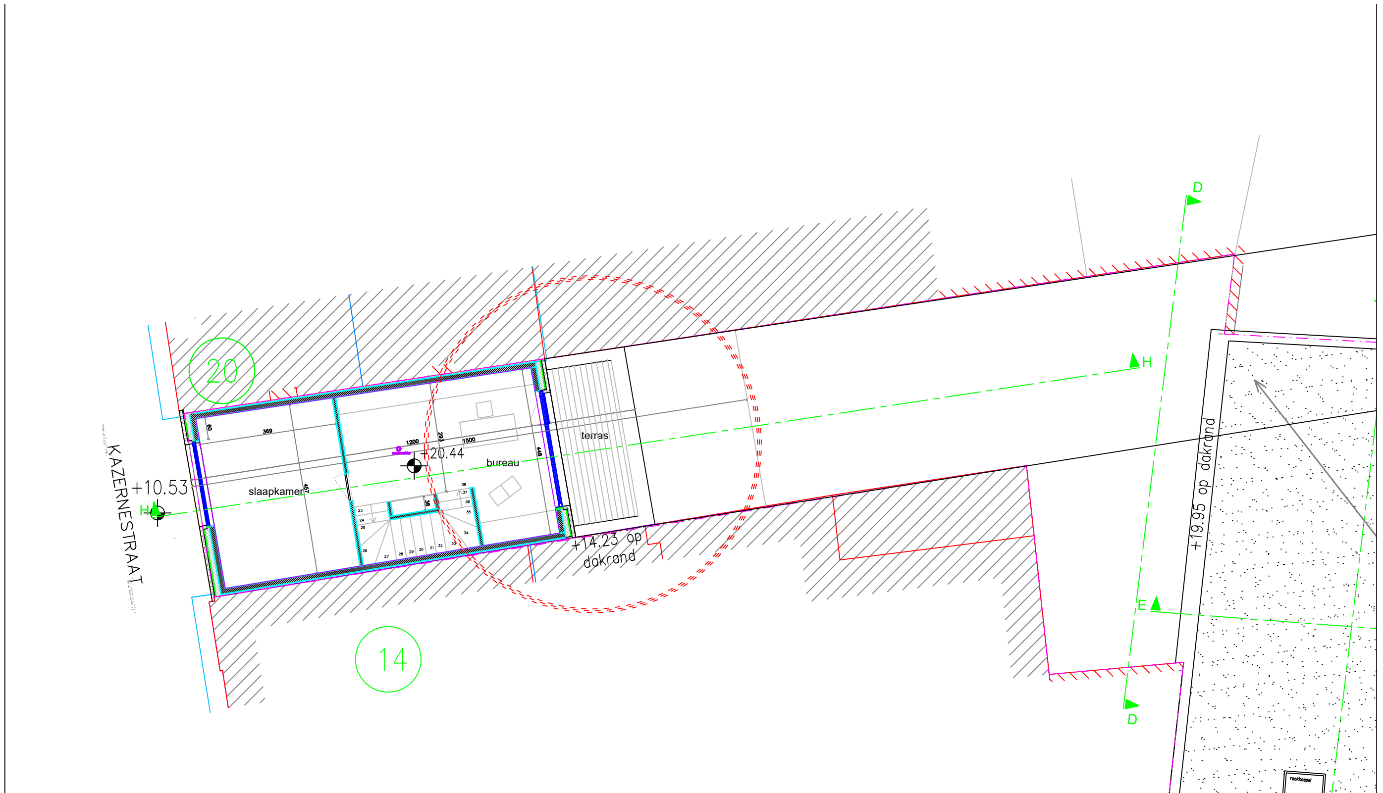
Bestaande toestand : Verdieping 03 1/100
