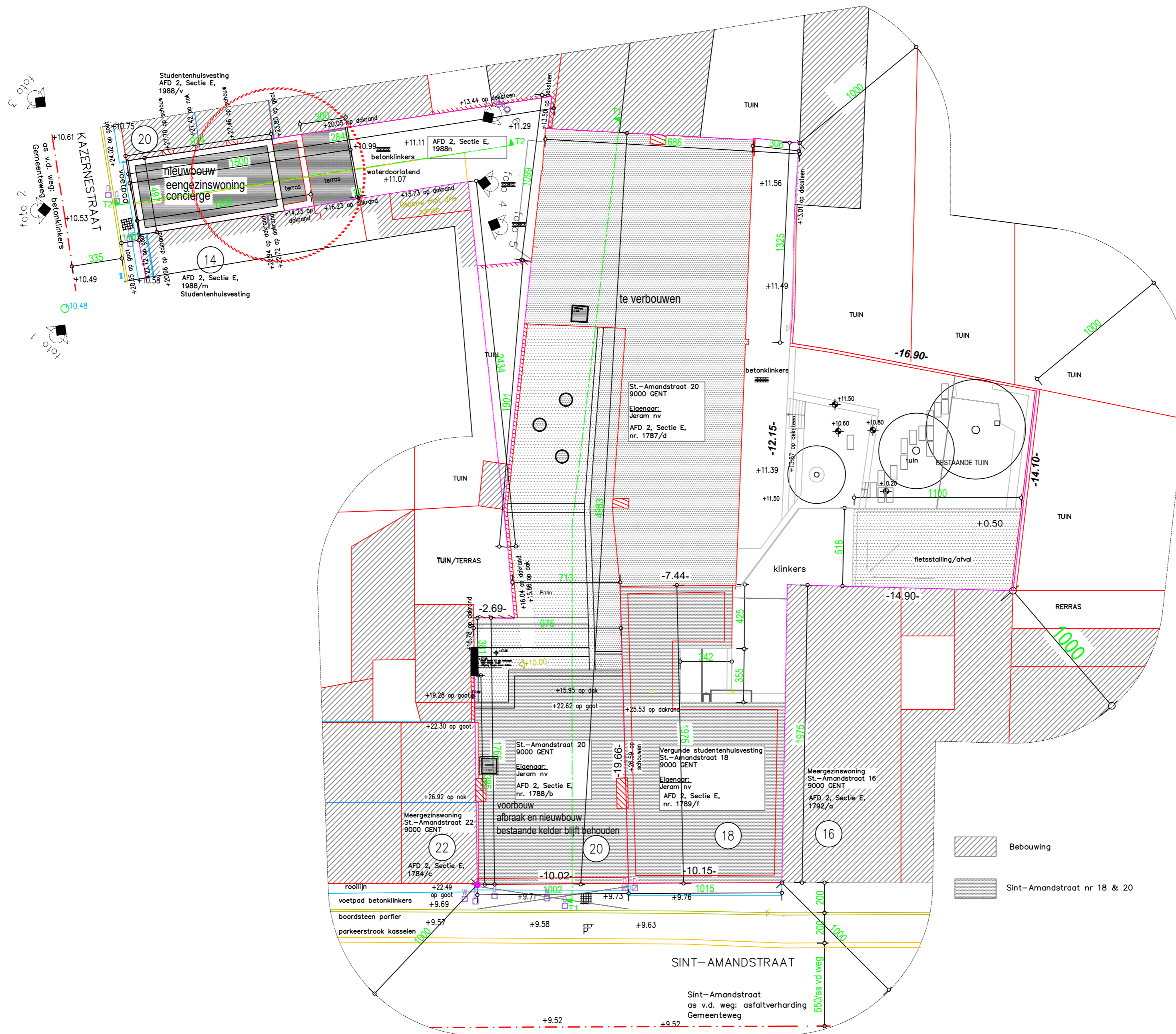
Bestaande toestand : Inplantingsplan 1/200
