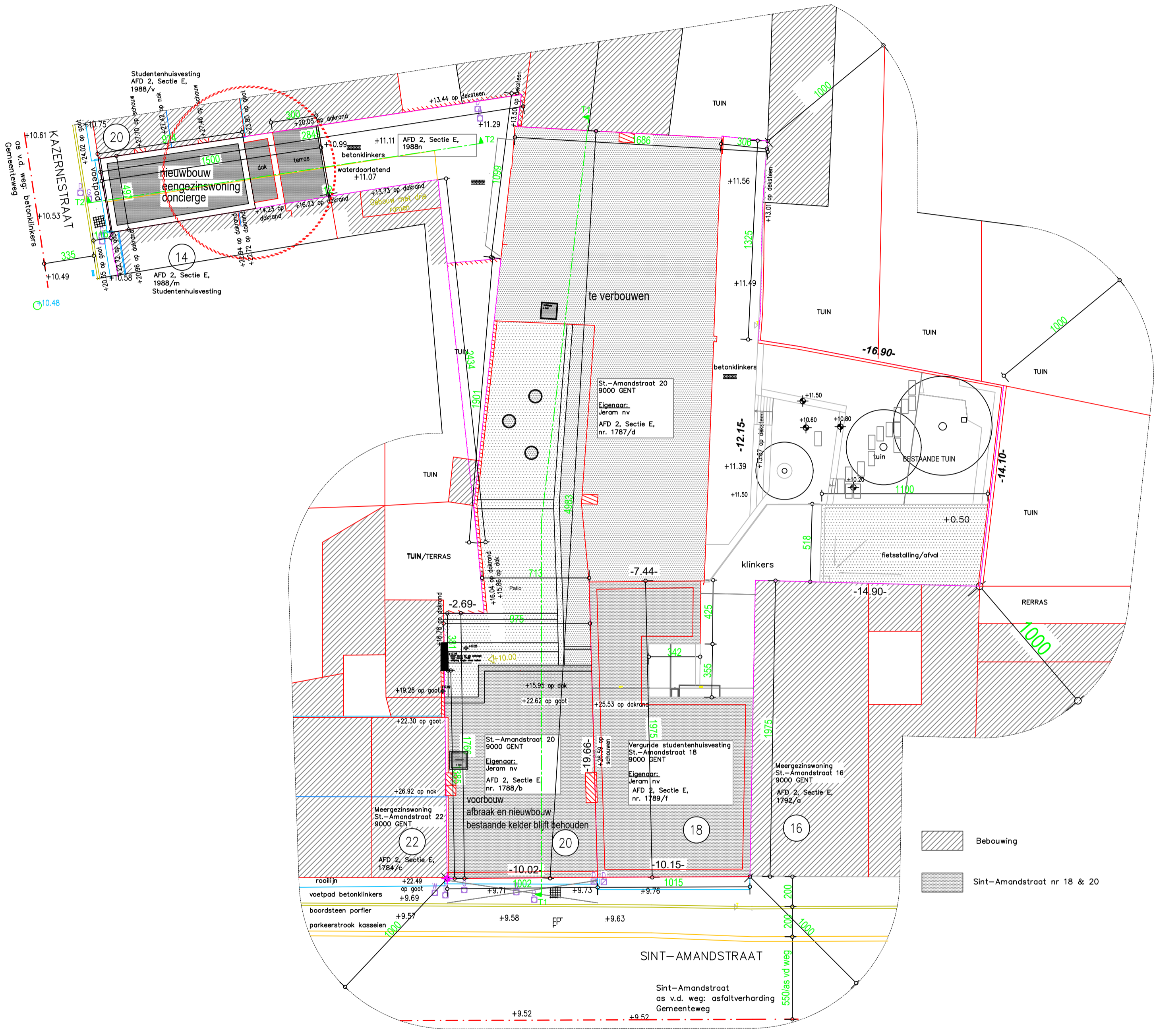
Vergunde toestand : Inplantingsplan 1/200
