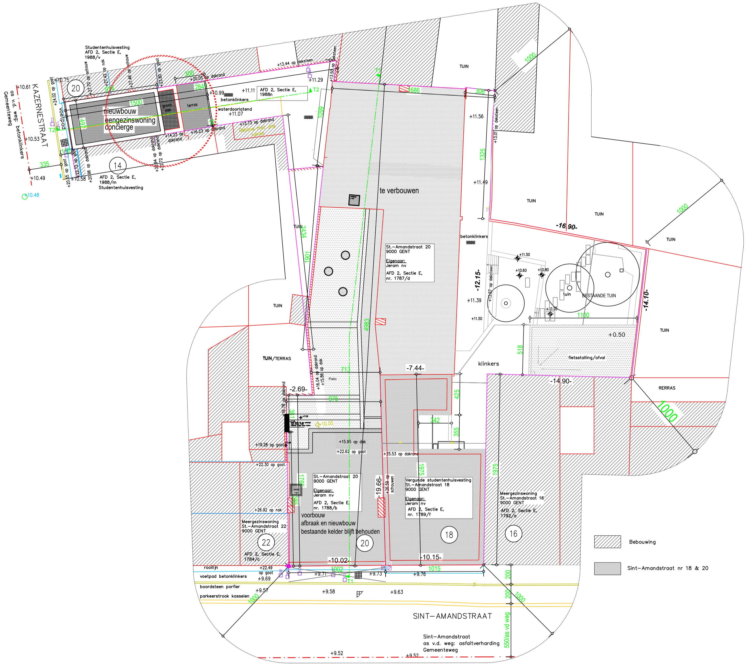
Nieuwe toestand : Inplantingsplan 1/200
